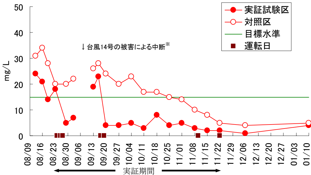
図8 隔離水界内の懸濁物質（SS）の経時変化
