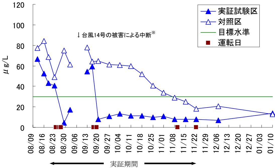
図7 隔離水界内のChl-aの経時変化
