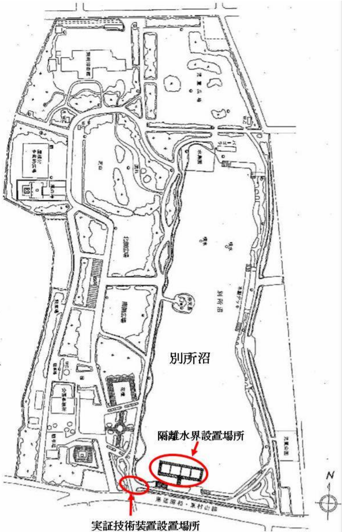
図5 別所沼における実験サイト（隔離水界）設置位置
