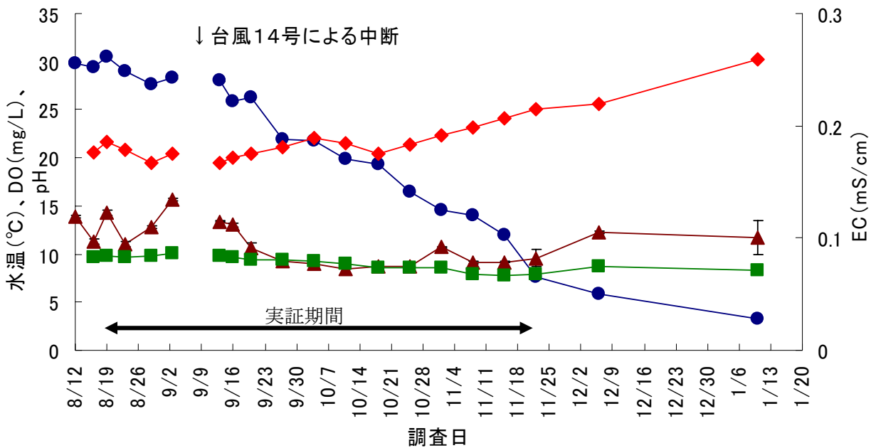
図11 対照区の表層（水深20cm）における水温、溶存酸素（DO）、pH及び導電率（EC）の経時変化（バーは標準偏差を表す）
