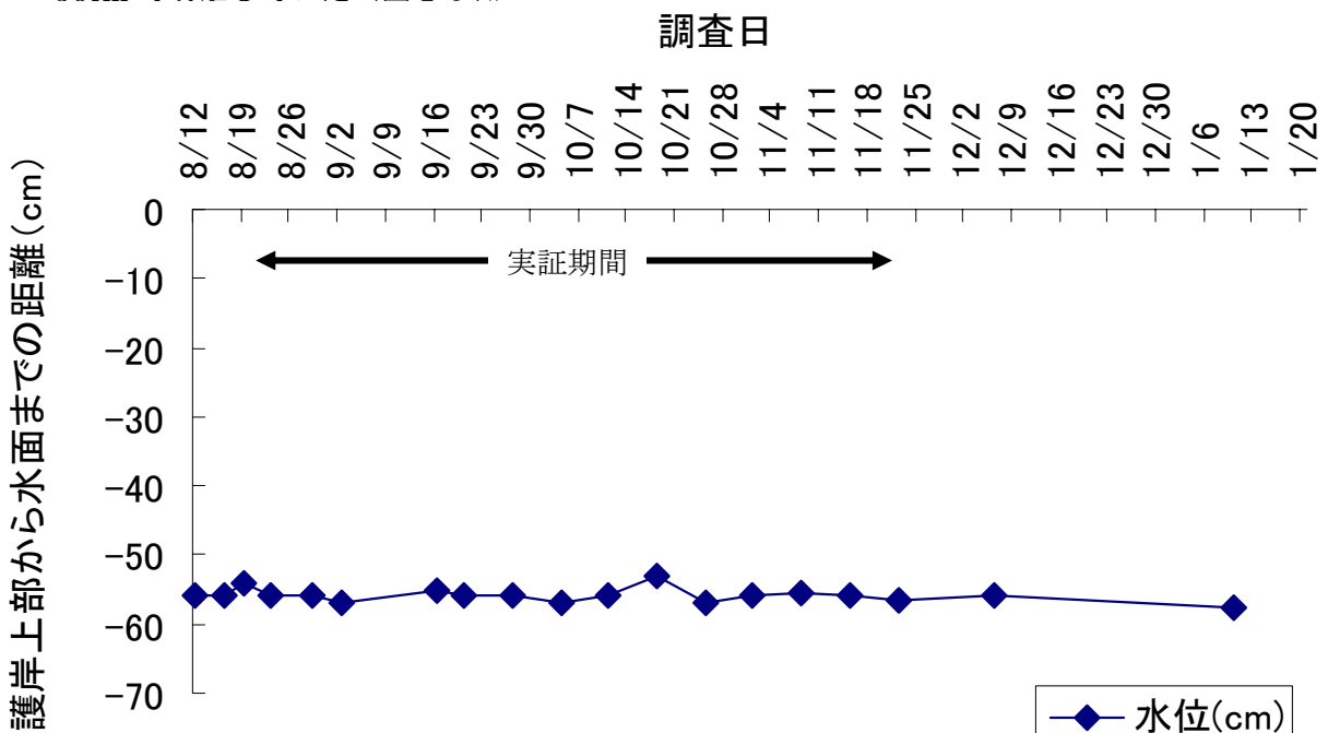
図19 別所沼における水位の変化
