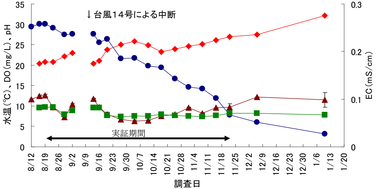
図10 実証試験区の表層（水深20cm）における水温、溶存酸素（DO）、pH及び導電率（EC）の経時変化（バーは標準偏差を表す）
