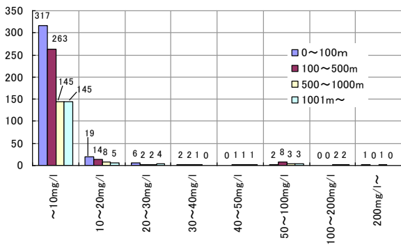
図7 【掘削深度別】温泉利用施設からの排水濃度(ほう素、ふっ素)
