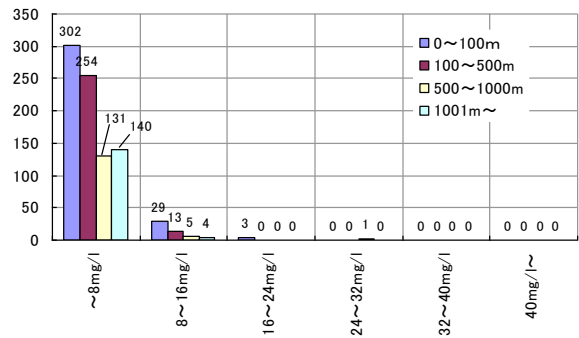
図7 【掘削深度別】温泉利用施設からの排水濃度(ほう素、ふっ素)
