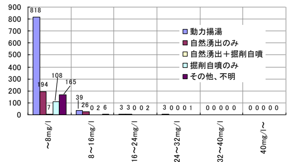
図6 【利用源泉形態別】温泉利用施設からの排水濃度(ほう素、ふっ素)
