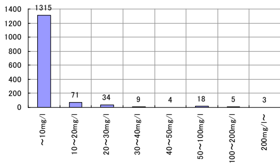
図5 温泉利用施設からの排水濃度(ほう素、ふっ素)
