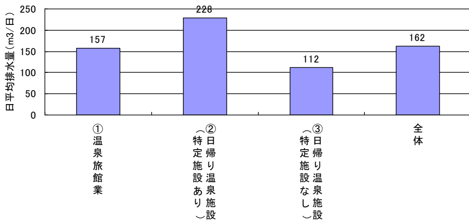
図4 温泉利用施設の日平均排水量(温泉利用施設の平均値)
