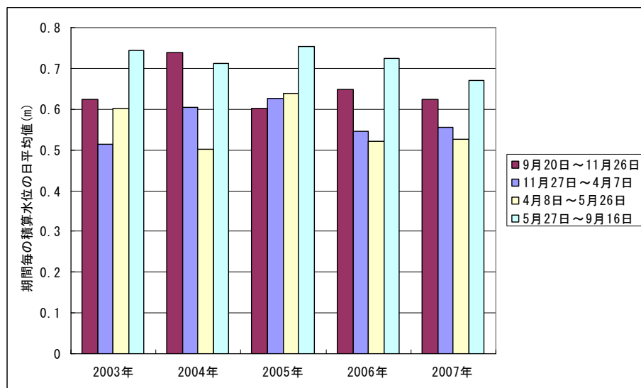
図 4.3-16 積算水位の時間変動
