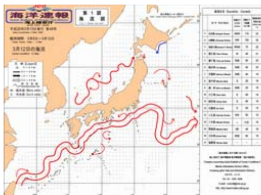
図 4.3-18(4) 日本近海の海流の時間変動
