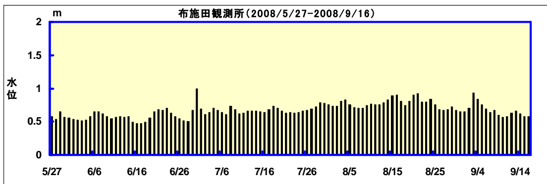
図 4.3-14 各クリーンアップ調査期間の水位の時系列
