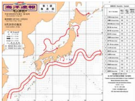
図 4.3-18(1) 日本近海の流れの時間変動
