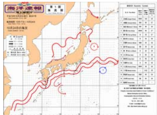
図 4.3-18(1) 日本近海の流れの時間変動
