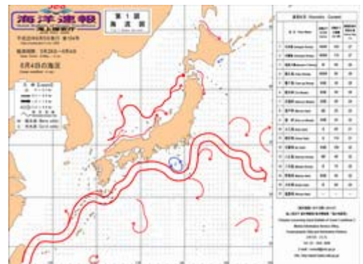
図 4.3-18(5) 日本近海の流れの時間変動
