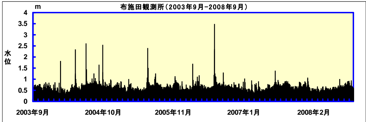
図 4.3-15 5年間の水位の時間変動
