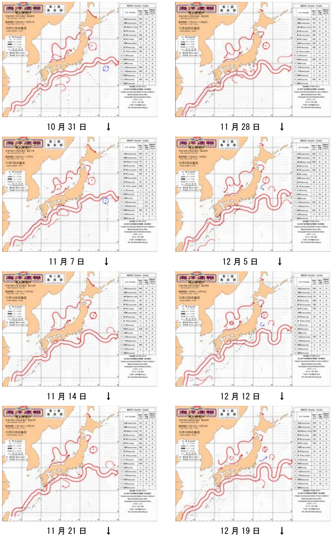
図 4.3-18 (2) 日本近海の流れの時間変動
