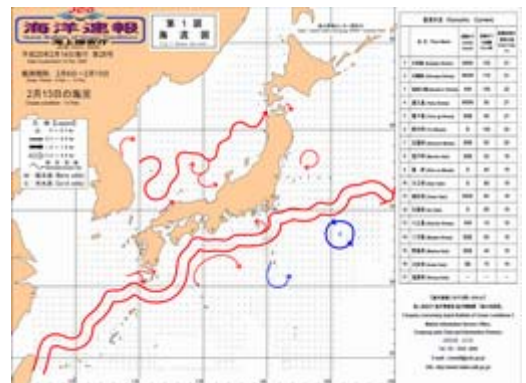
図 4.3-18(3) 日本近海の流れの時間変動
