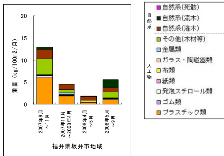
図 4.3-17 第 1 回～第 6 回までの共通調査における漂着ゴミの重量の推移
