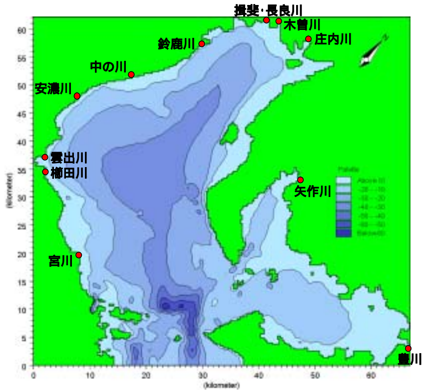
図 5.3-1 伊勢湾の海底地形
