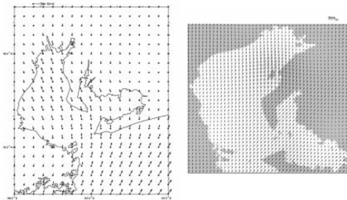
図 5.3-6 風データの比較
