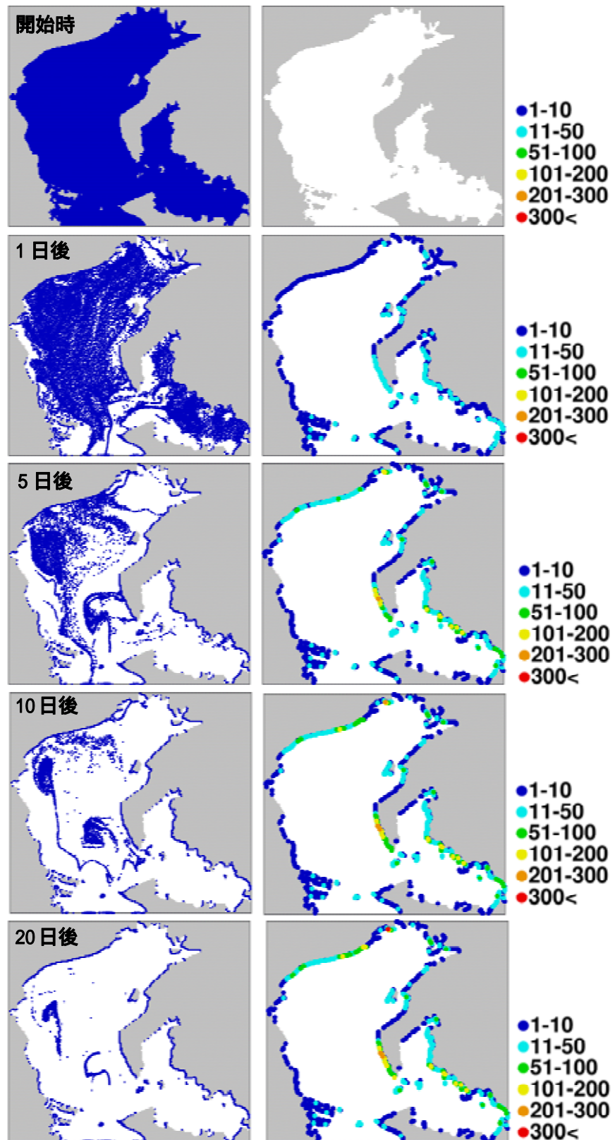
図 5.3-27 伊勢湾全域に漂流物を置いたケース（ペットボトルを想定） （左図：漂流物の分布、右図：漂着量）
