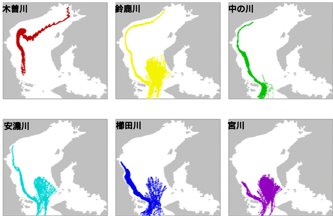
図 5.3-26 風の影響なしのケースの計算結果
