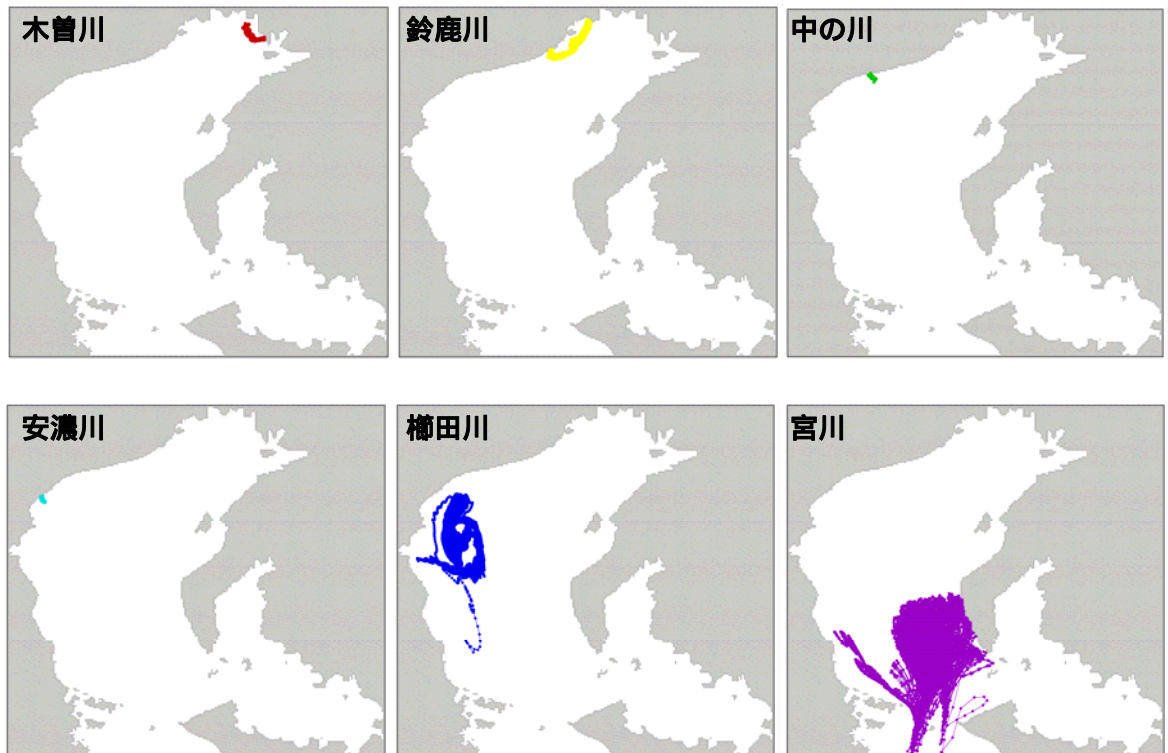
図 5.3-25 ペットボトルを対象とした漂流経路の計算結果
