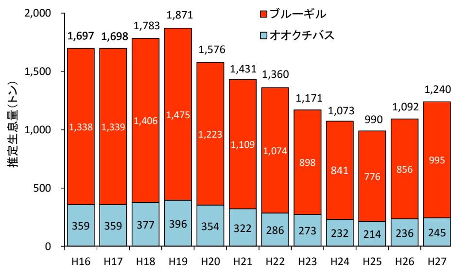
主な外来魚の推定生息量
