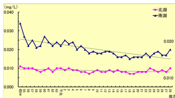
全りん*の経年変化
