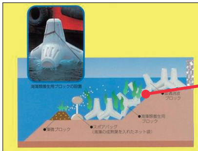
関西国際空港の緩傾斜護岸と藻場の再生
