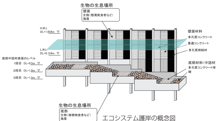
エコシステム護岸の概念図
