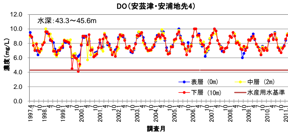
図2.9-2(2) DOの経年変化（湾外：安芸津・安浦地先4）
