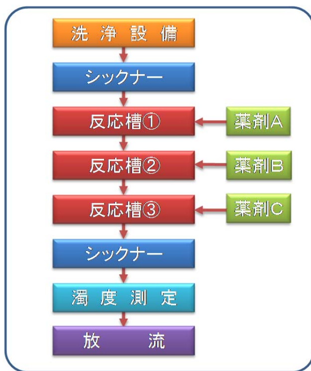
図 2.1.3-6 洗浄処理における汚水処理フロー図の例
