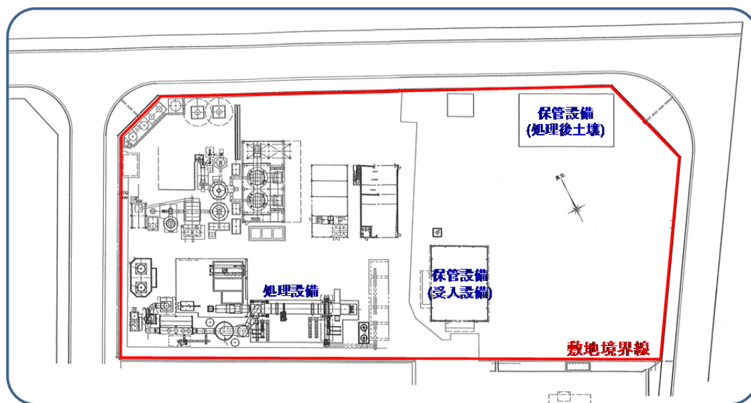
図 2.1.3-3 施設配置図の例
