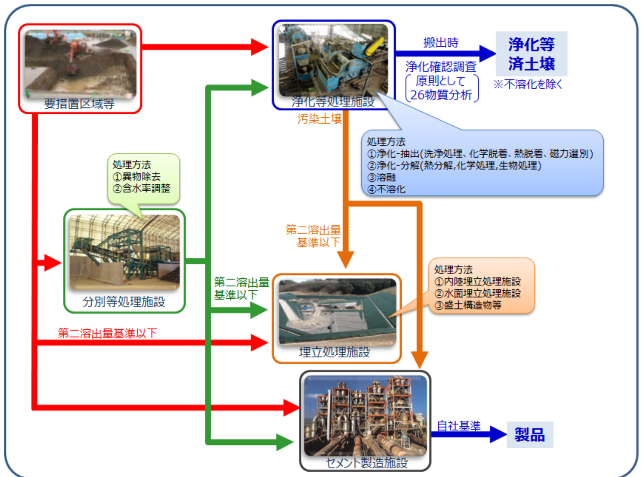
図 1.5.2-1 要措置区域等から搬出される汚染土壌の流れ
