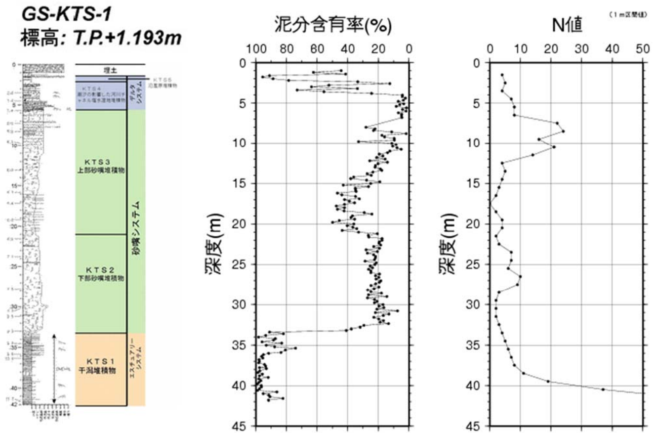
図-20 地質柱状図の一例
