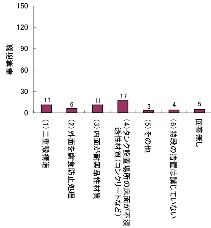
【「地下」に設置されたタンク】
