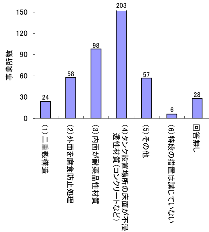
【「地上」に設置されたタンク】
