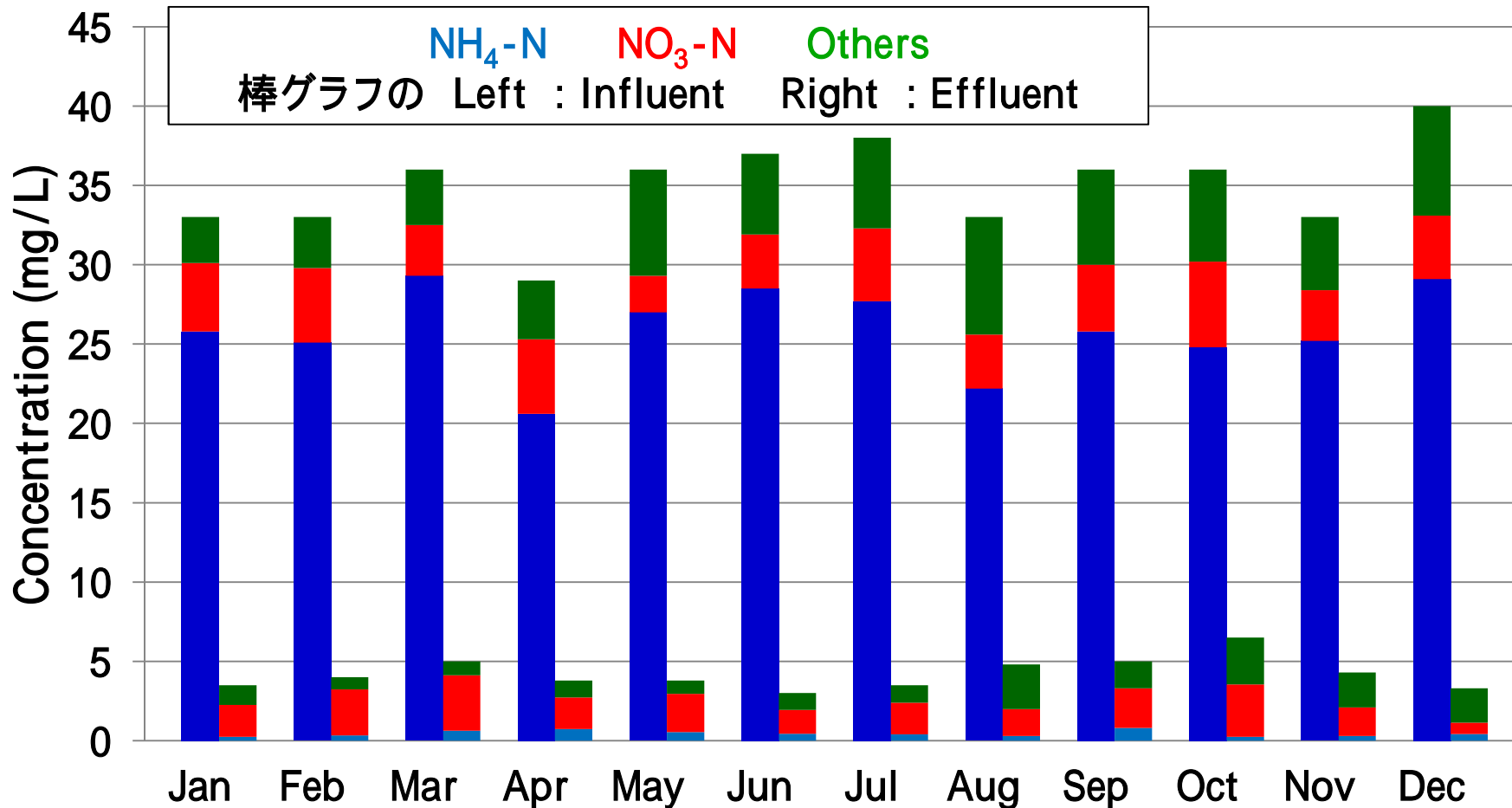
ビズン処理場における原水と処理水の窒素組成 (2015年)
