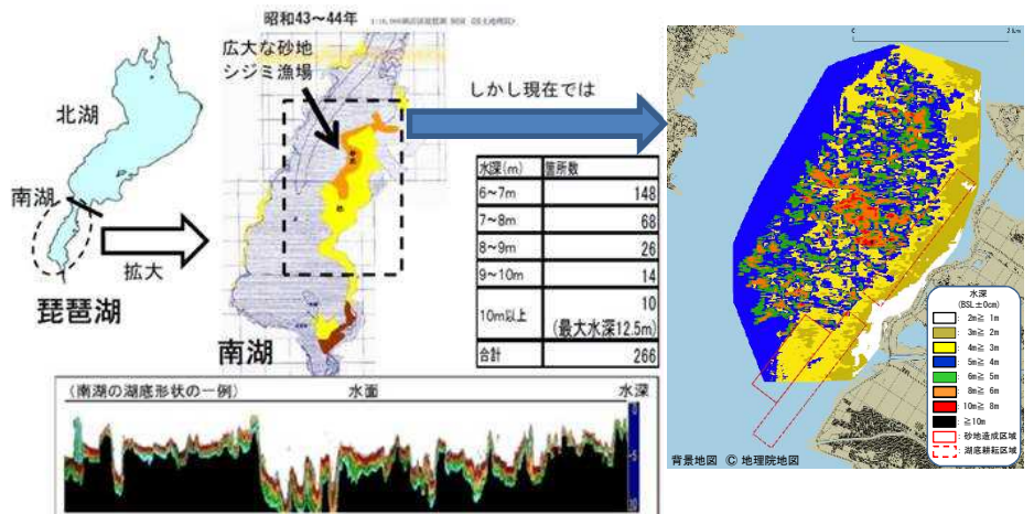
【図表5】南湖の湖底環境
