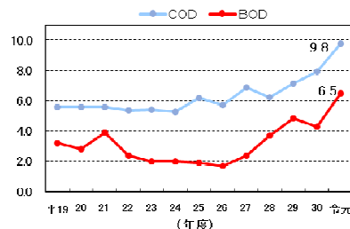
【図表3】西の湖BOD・COD経年変化
