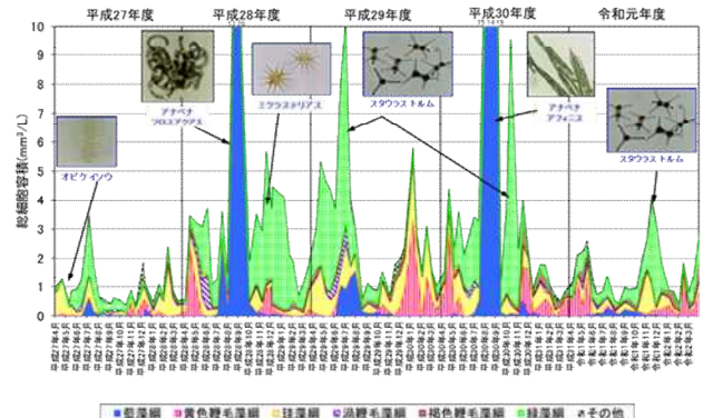
【図表13】南湖唐崎沖中央における植物プランクトンの総細胞容積の経月変動（表層）
