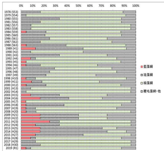
【図表12】植物プランクトンの種構成の変化
