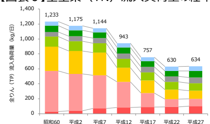
【図表7】全りん（TP）流入負荷量の経年変化
