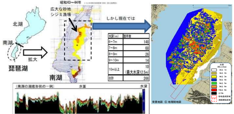
【図表5】南湖の湖底環境
