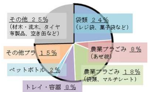
琵琶湖のプラスチックごみ実態把握調査（令和元年6月赤野井湾）
