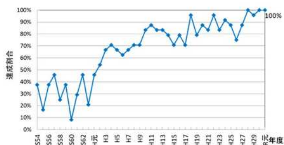
県内河川の環境基準（BOD）の達成率
