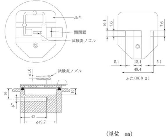
図 セタ密閉式引火点測定器の試料カップ
