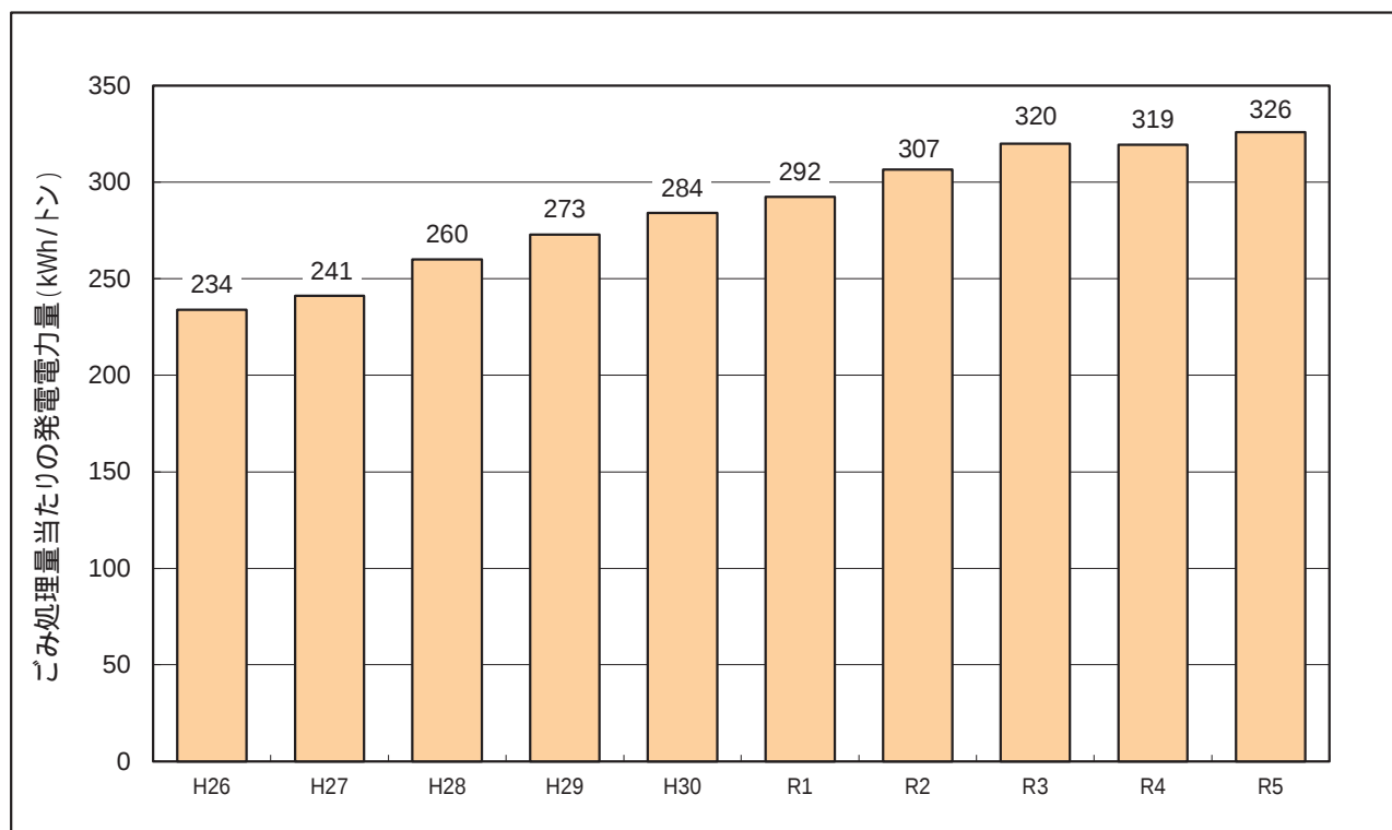
図 - 13 ごみ処理量当たりの発電電力量 注14)
