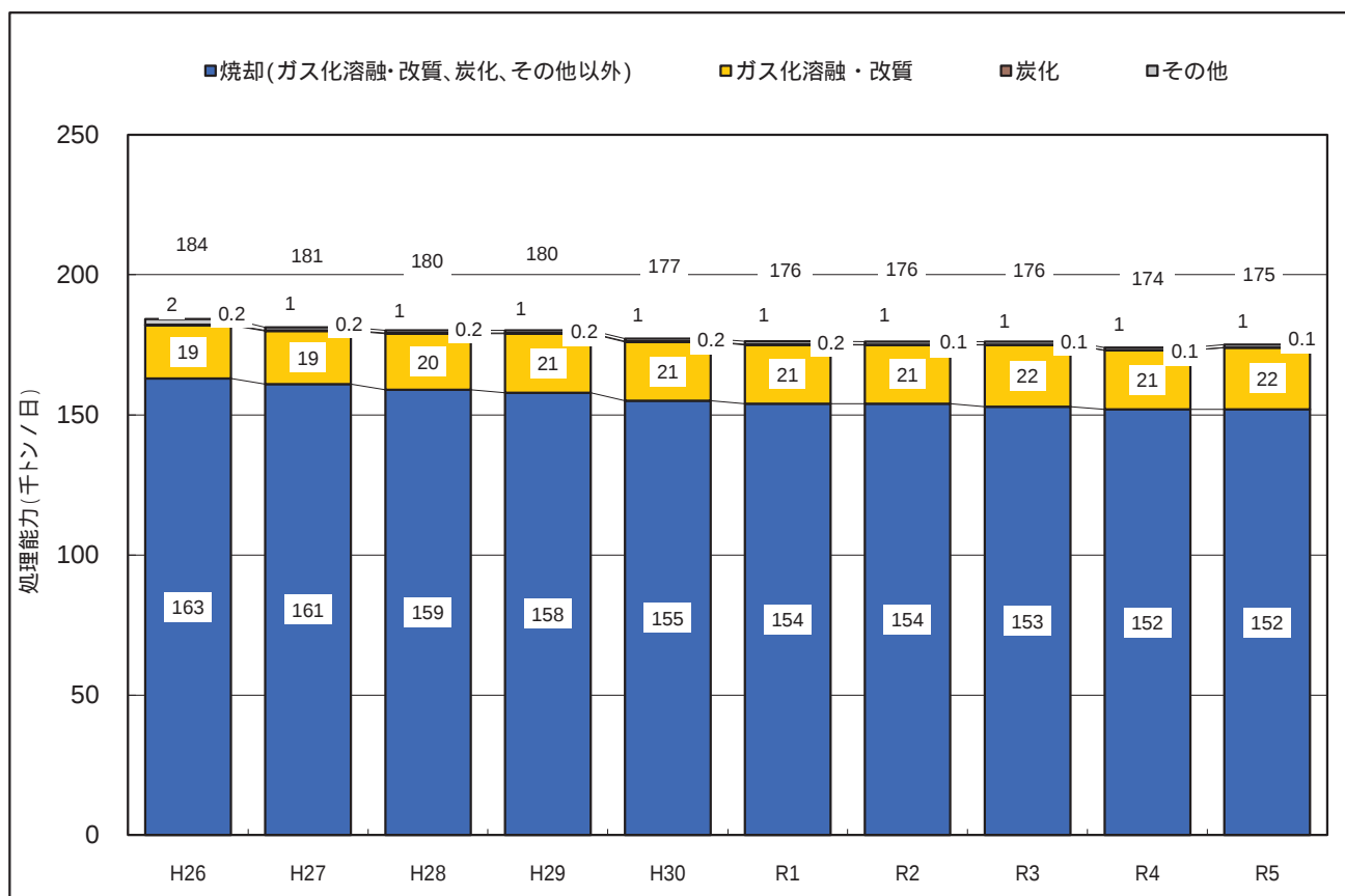
図 - 1 0 ごみ焼却施設の種類別処理能力の推移
