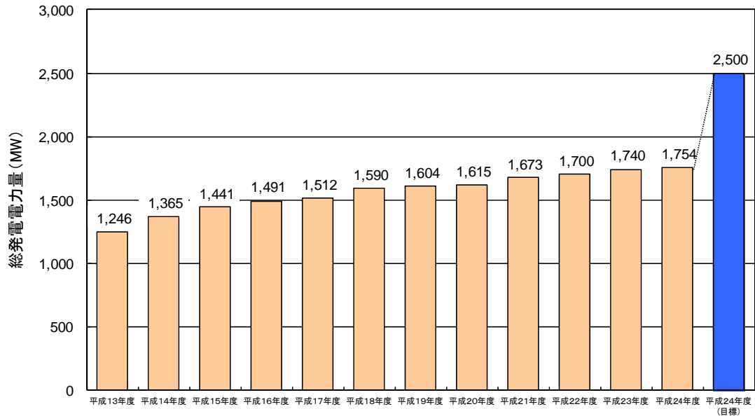
図-17 総発電能力の推移
