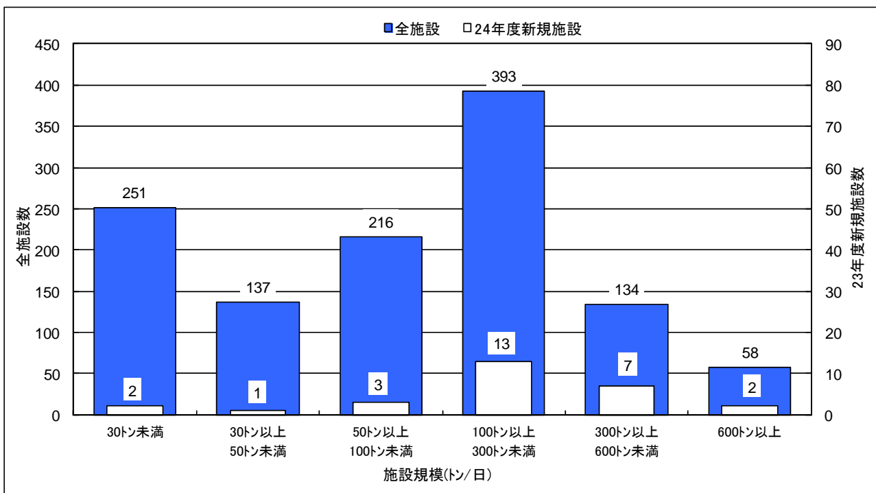
図-11 ごみ焼却施設の規模別施設数
