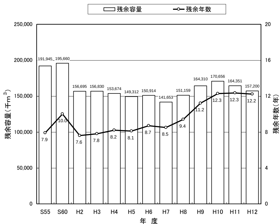
図－１６ 残余容量と残余年数の推移
