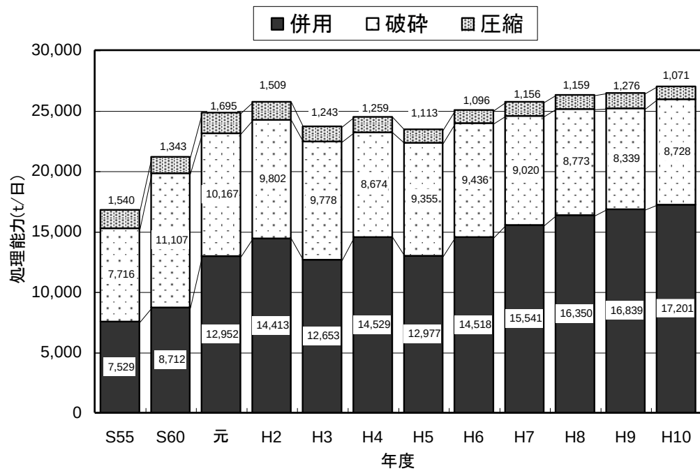
図－１３ 粗大ごみ処理施設能力の推移
