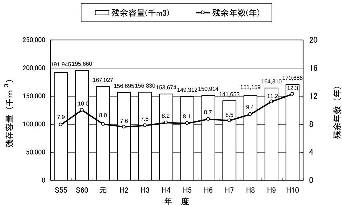
図-15 残存容量と残余年数の推移
