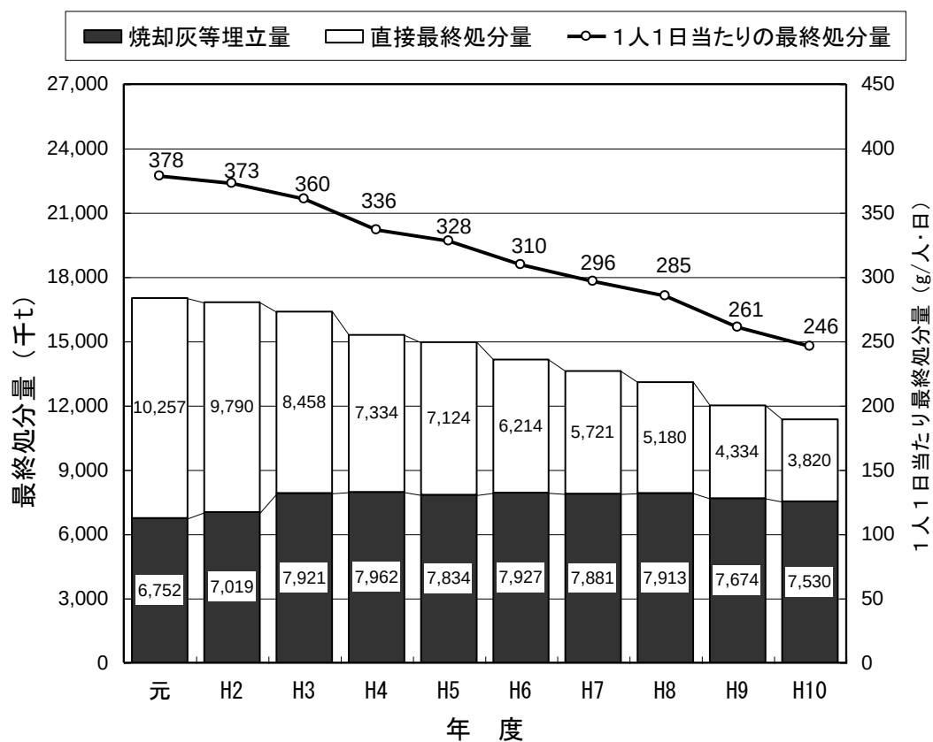
図－8 最終処分場と1人1日当たり最終処分量の推移
