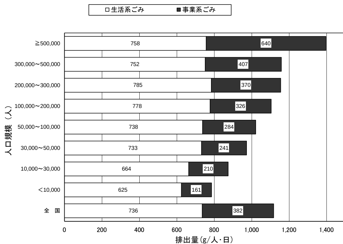
図ー4 人口規模別1人1日当たりごみ排出量（平成10年度実績）
