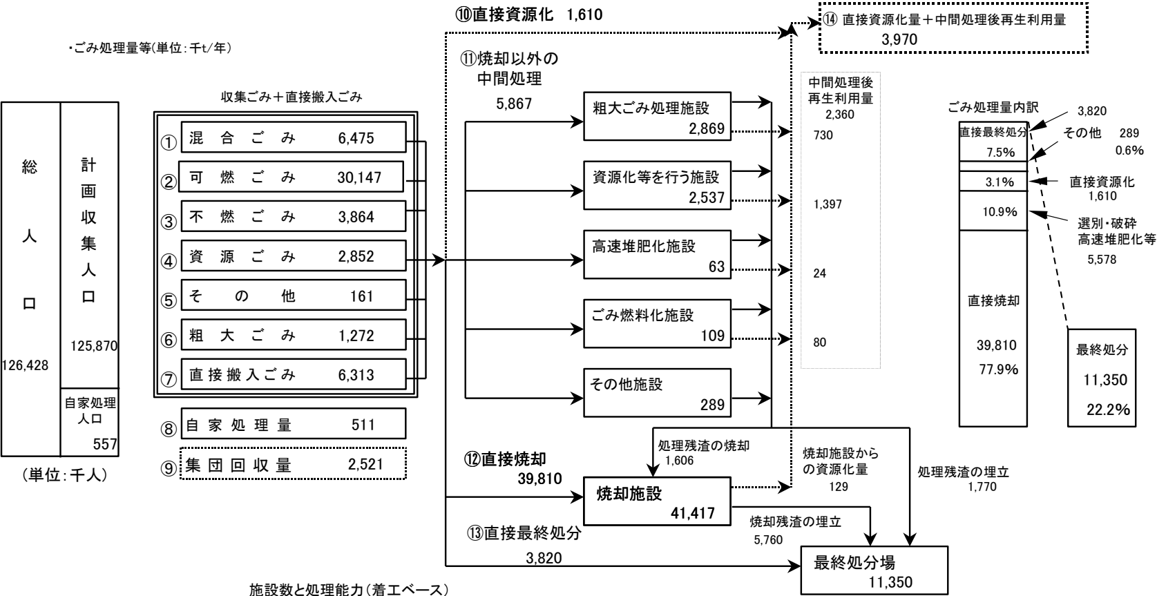
施設数と処理能力(着工ベース)
