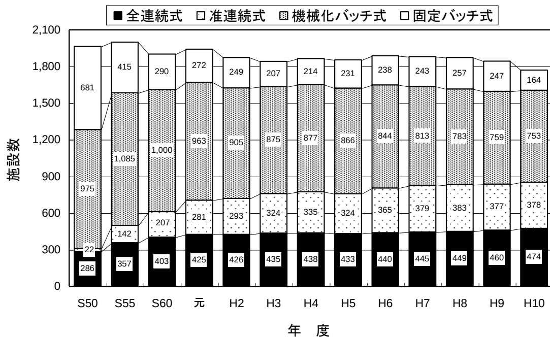
図-9 ごみ焼却施設数の推移
