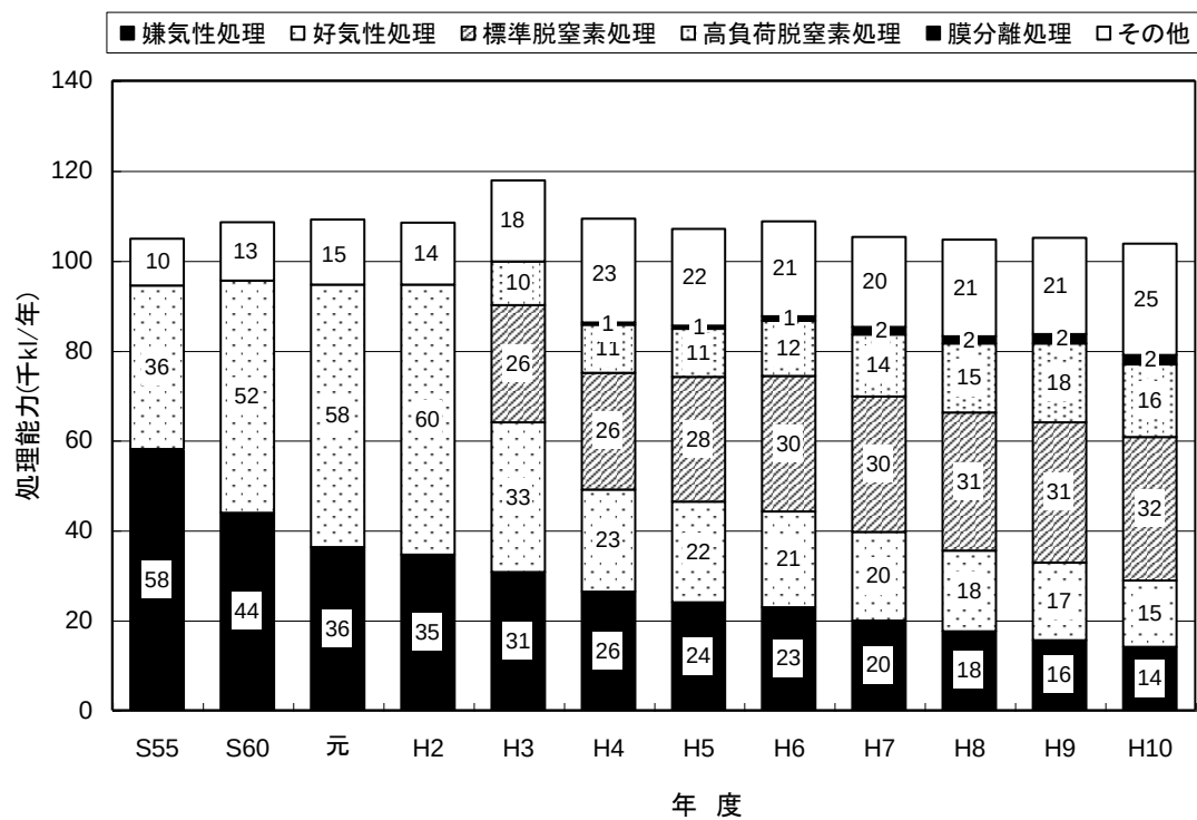
図－２８ し尿処理施設処理能力の推移
