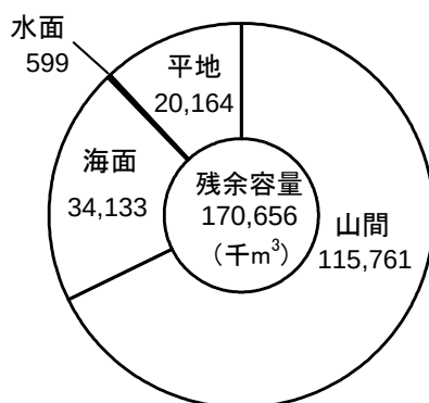
図-17 市町村・事務組合設置の最終処分場の残余容量の内訳（設置場所別）
