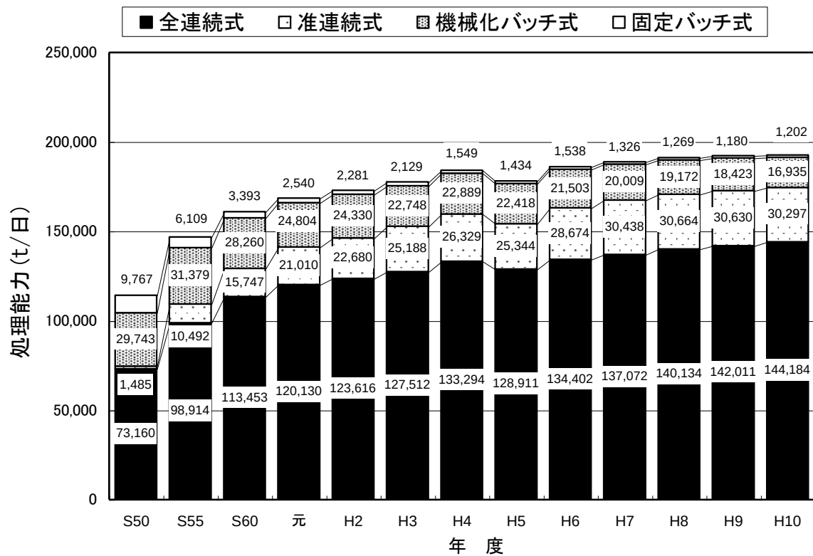
図－１０ ごみ焼却施設炉形式別能力の推移
