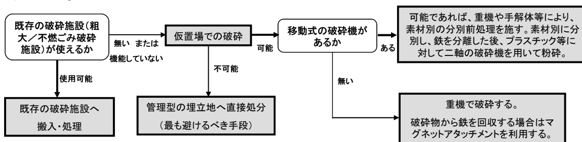
図 リサイクルが見込めない場合の処理方法
