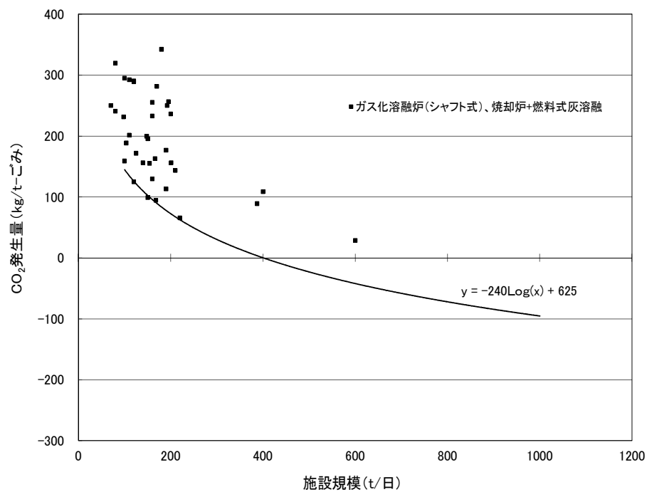
図 参-4 基幹的設備改良の CO 2 排出量基準値 (分類 1)
