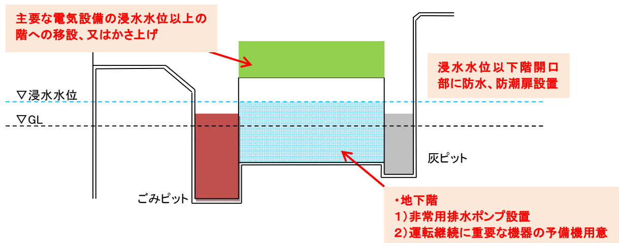
図 I .2.1 浸水対策の一例
