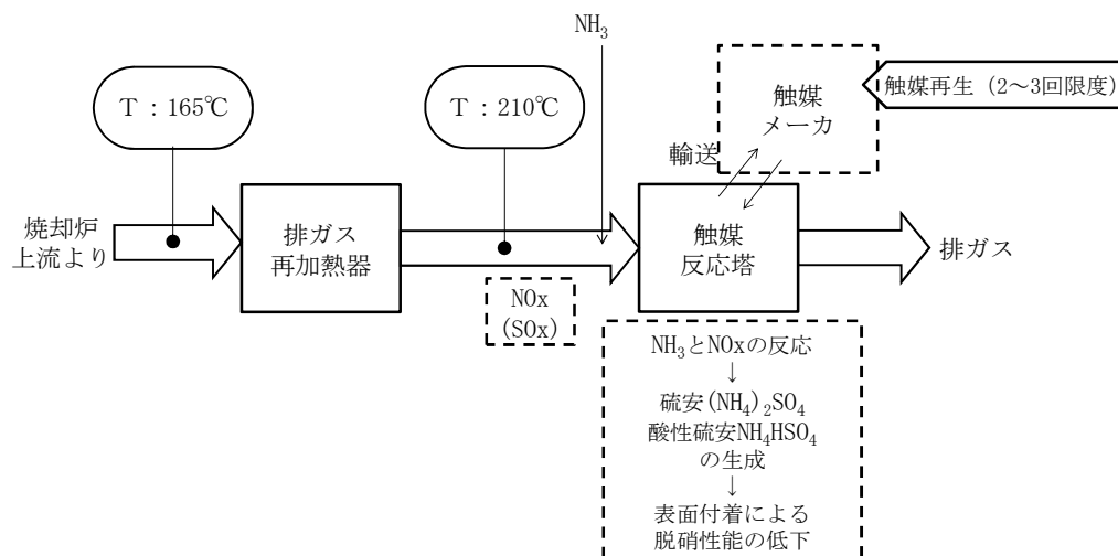
図 I.3.6 触媒脱硝フロー（例）
