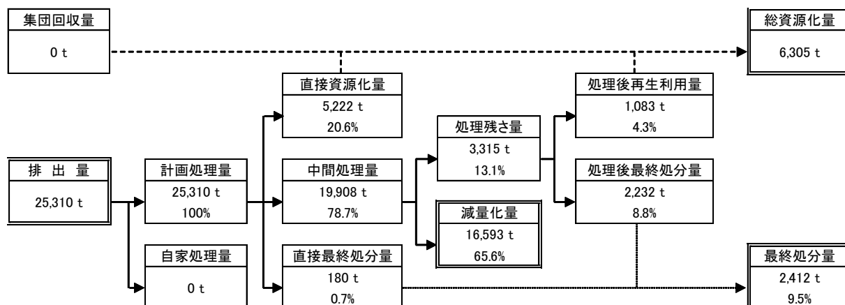
図3 目標達成時の一般廃棄物の処理状況フロー (令和2年度)
