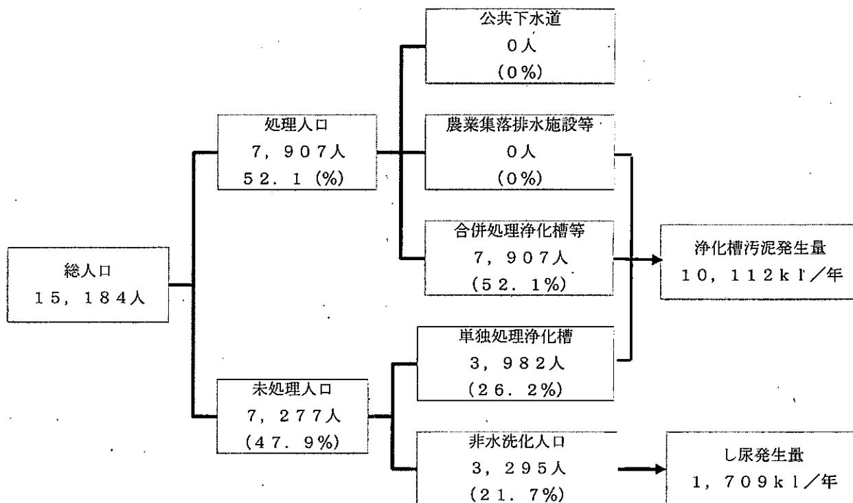
生活排水の処理状況フロー
