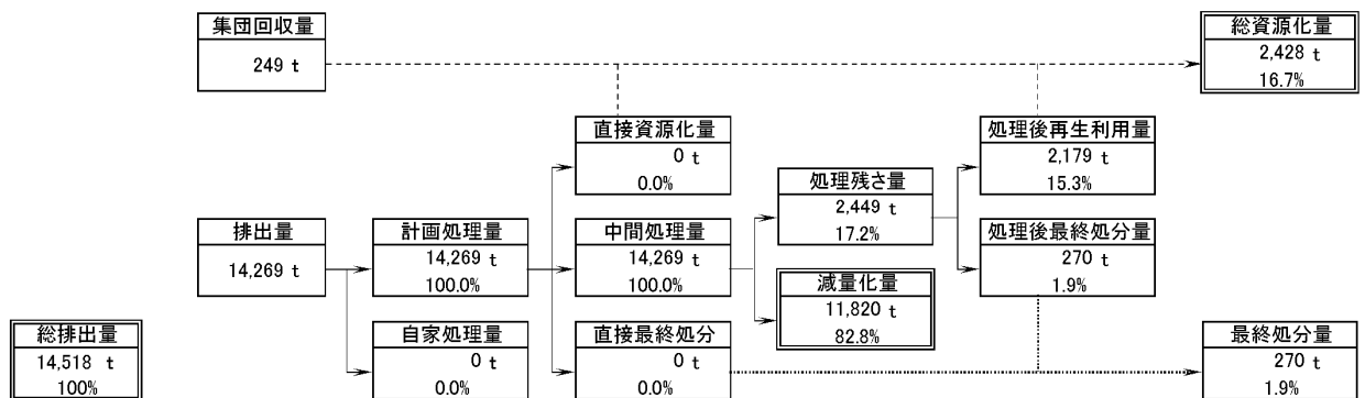
図4 目標達成時の一般廃棄物の処理状況フロー(R4)
