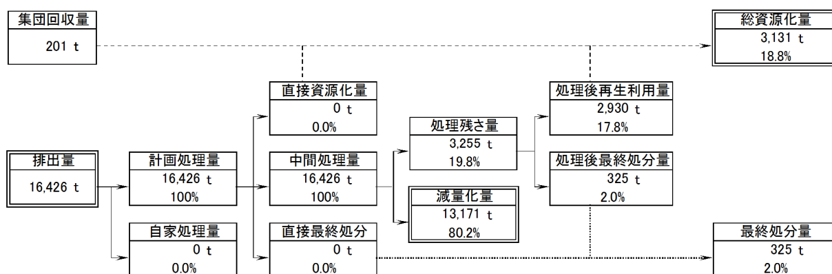
図 2 一般廃棄物の処理状況フロー(H26)
