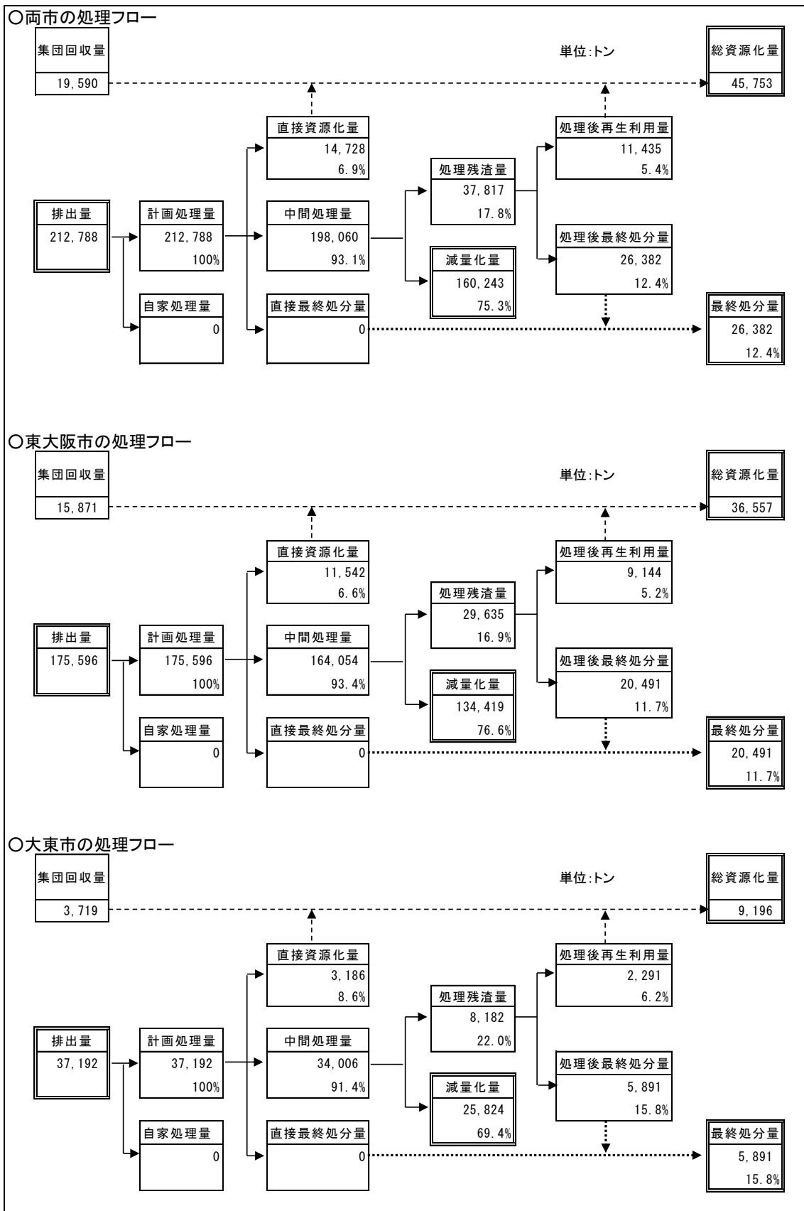
図4 目標達成時の一般廃棄物の処理フロー
