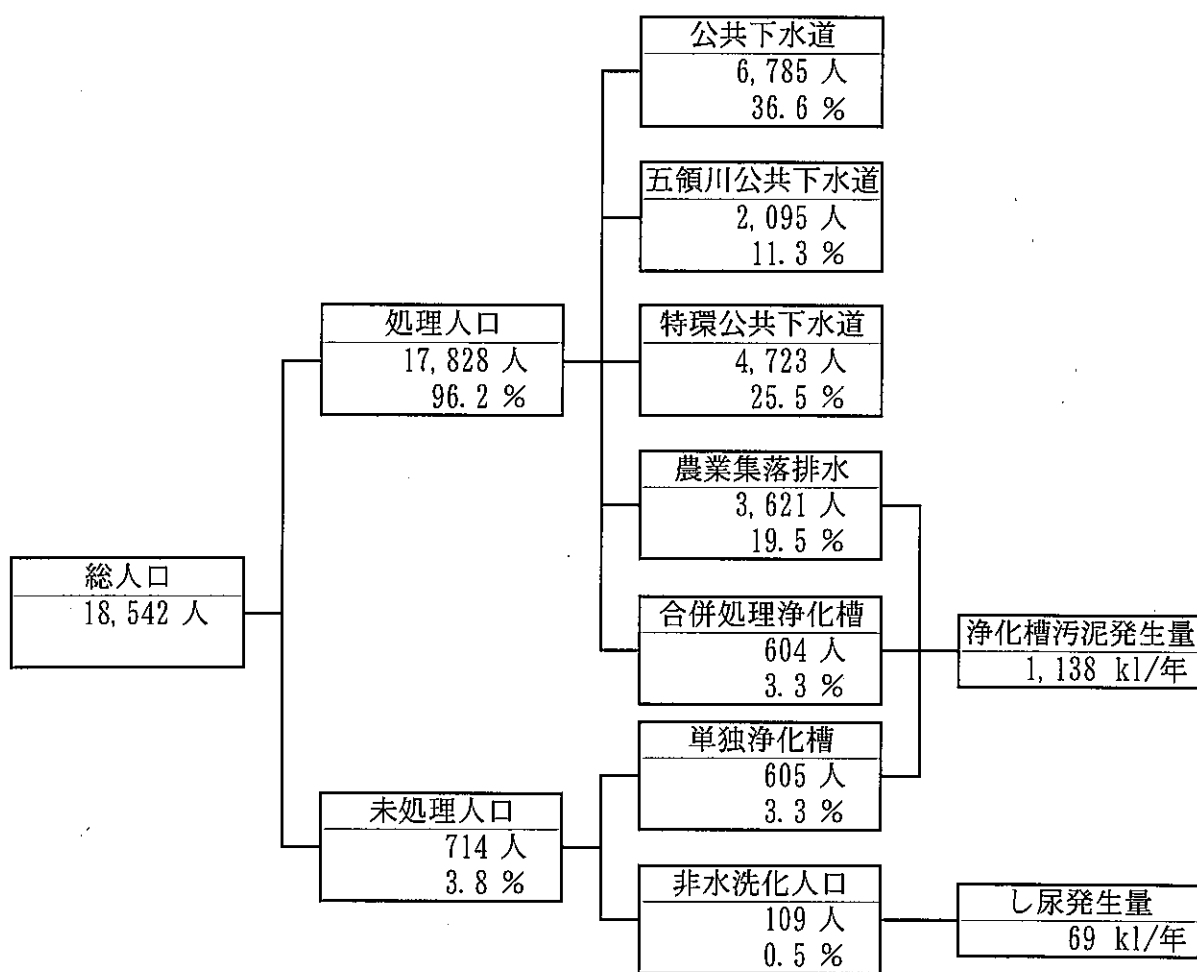
図1 生活排水の処理状況フロー
