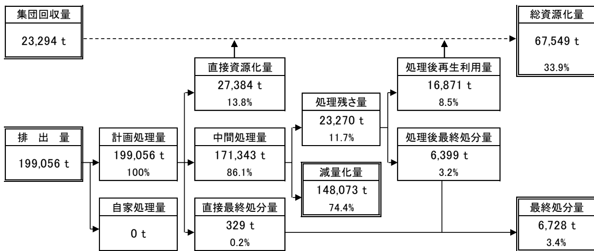
図-3 目標達成時の一般廃棄物（ごみ）の処理状況フロー（平成34年度）
