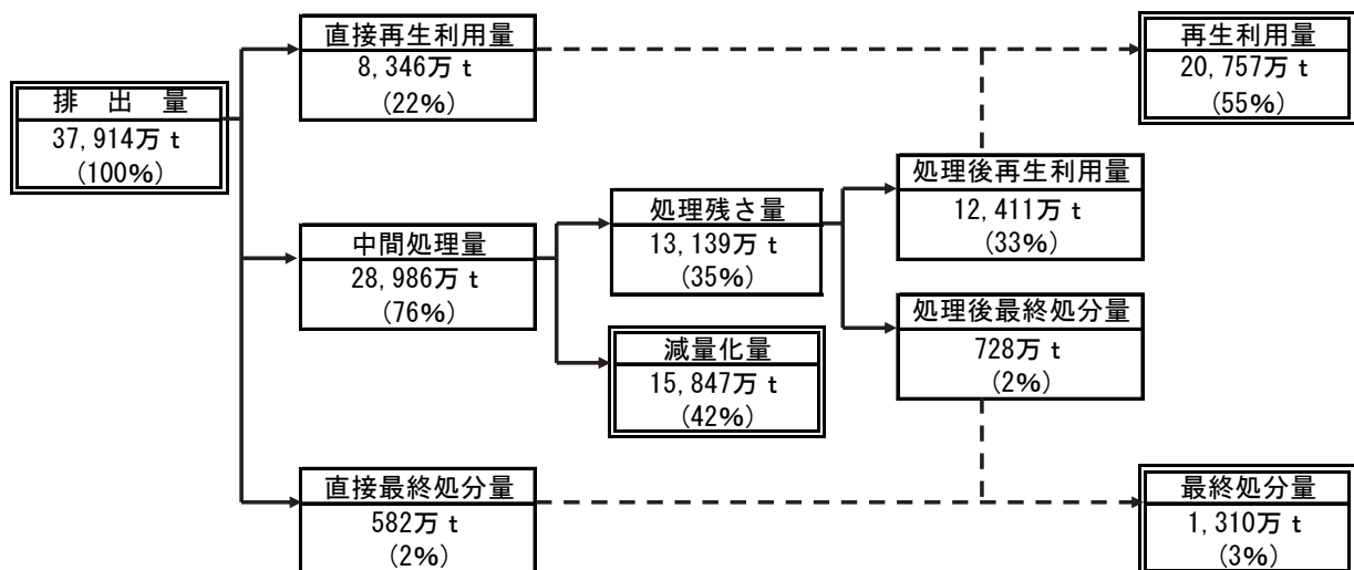
図 3-1-1 産業廃棄物の処理・再資源化の流れ（平成 24 年度）
