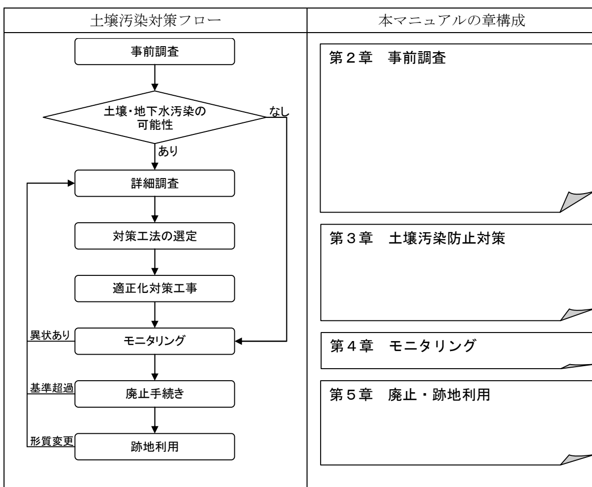
図 1-2 土壌汚染対策フロー
