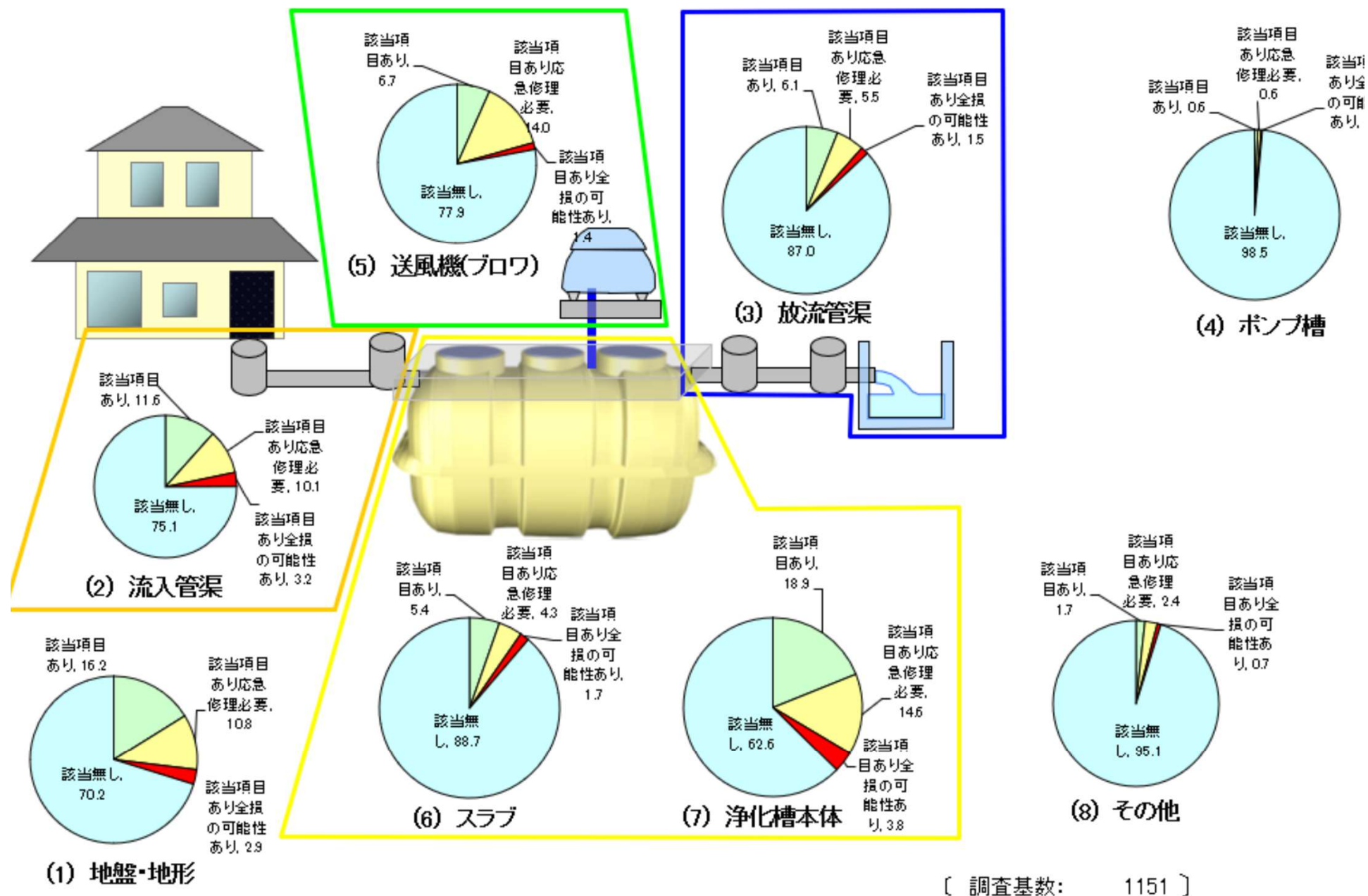
東日本大震災における浄化槽の被災状況 (大項目の該当施設の割合 %)
