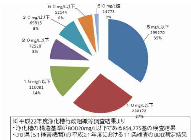
○図3 浄化槽の処理水質
