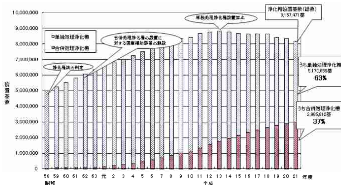
○図1 浄化槽の整備の状況と経緯
