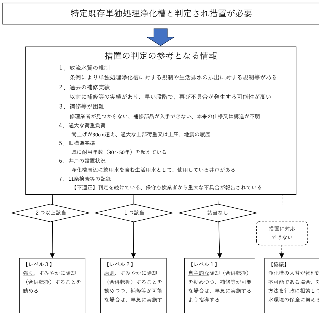
図4. 1 特定既存単独処理浄化槽の判定フロー（例）
