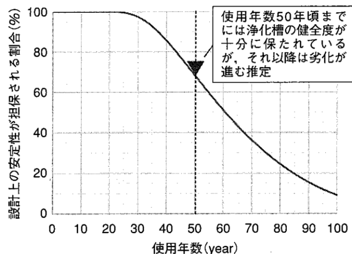
図4. 2 設計上の安全性が担保される割合の推移 6)
