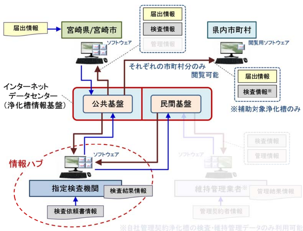
図 7.3 宮崎県における当面の浄化槽台帳システム導入・運用方法
