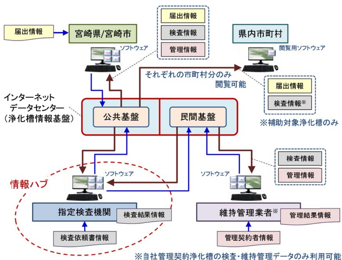
図 7.4 宮崎県における将来的な浄化槽台帳システム導入・運用方法
