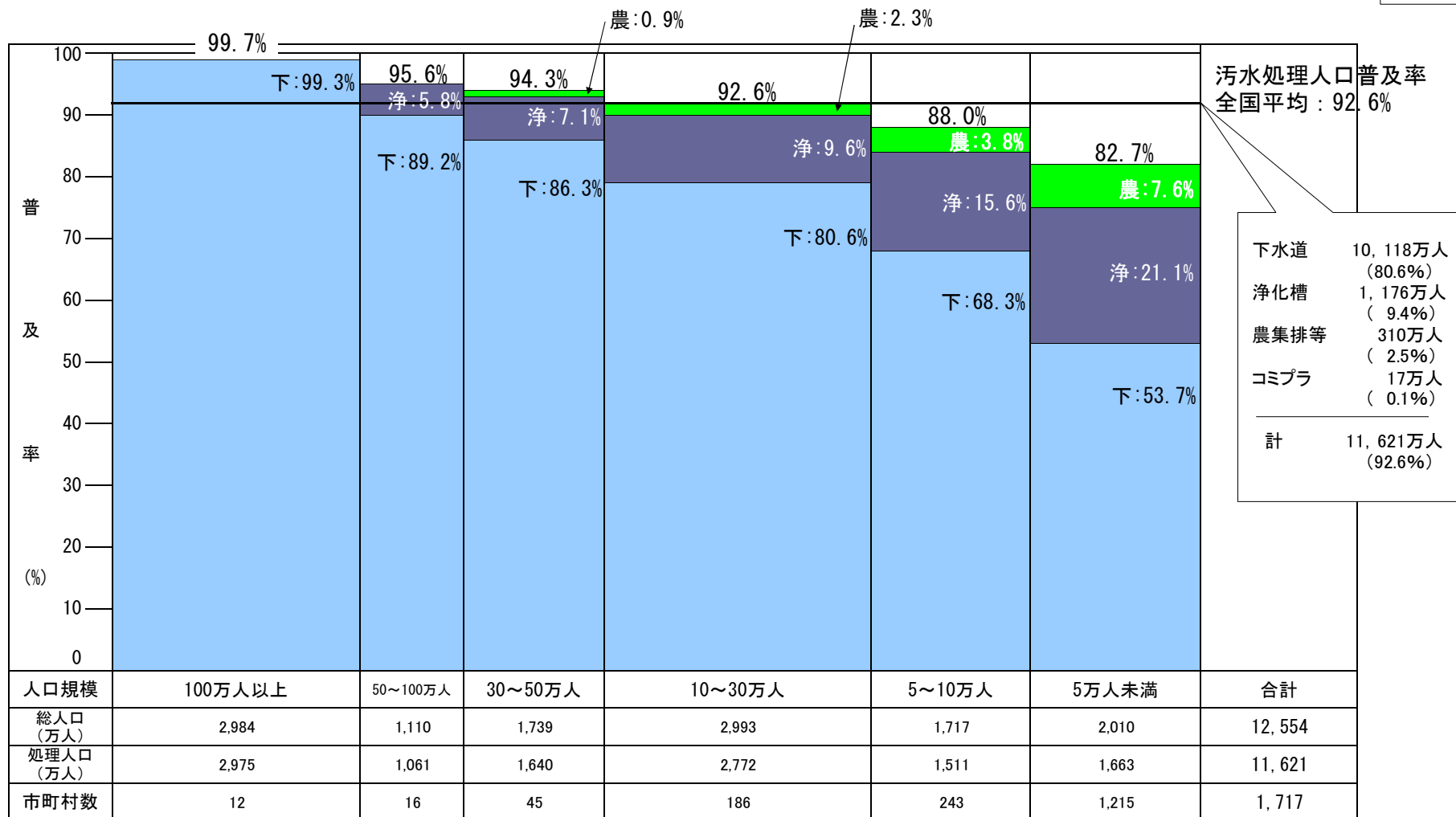
○都市規模別汚水処理人口普及率（令和3年度末）
