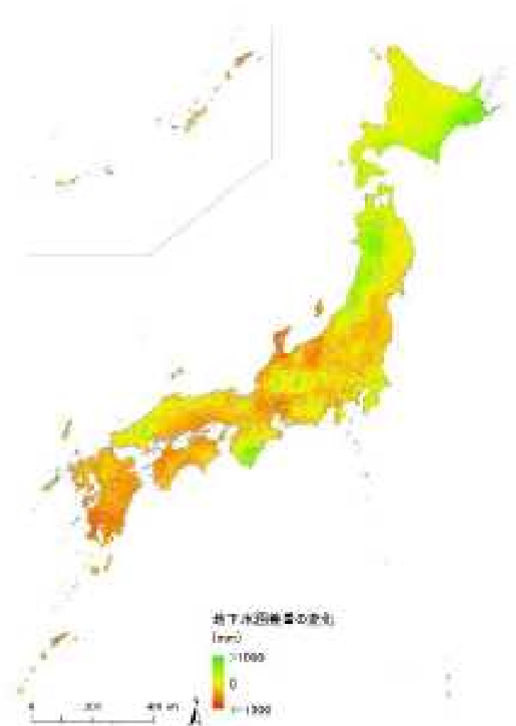
図 III-12 地下水涵養量の変化 (1976 年と 2009 年の比較)
