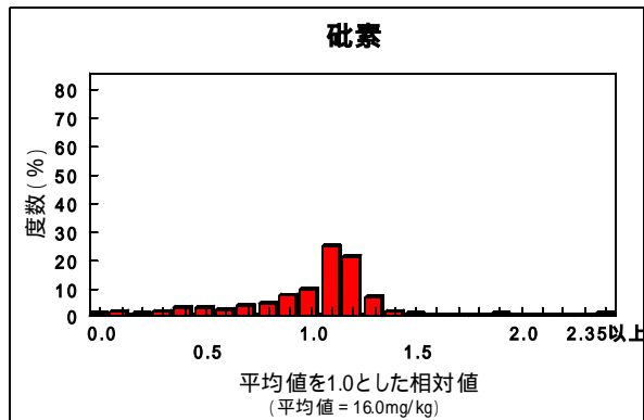
図1 廃棄物試料のヒストグラム (重金属類)
