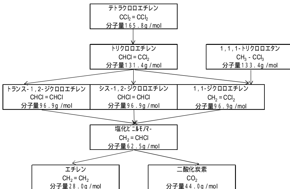
図：塩化ビニルモノマーの主な分解経路 12)
