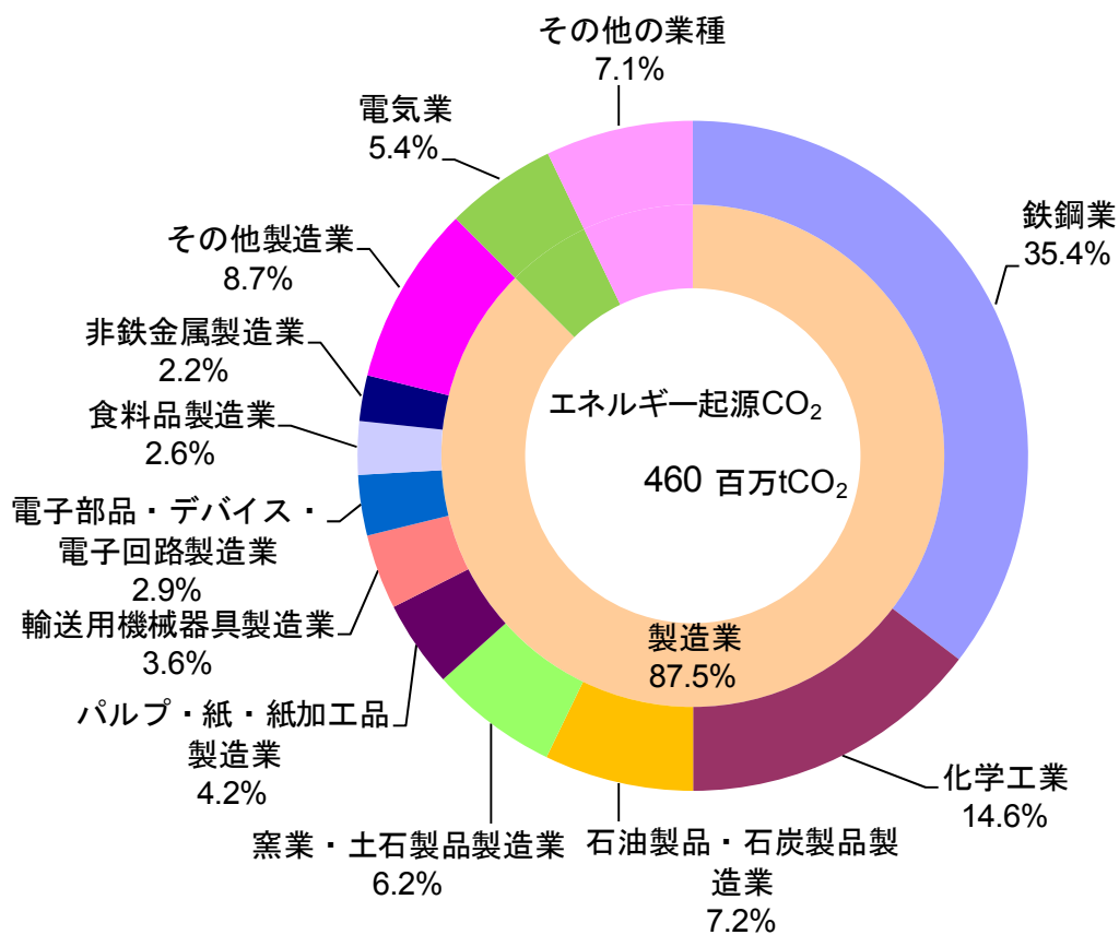
図 3-16 エネルギー起源 CO 2 【特定事業所】
