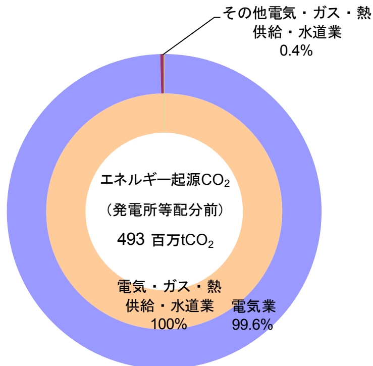
図 3-2 4 エネルギー起源 CO 2 (発電所等配分前)【特定事業所】
