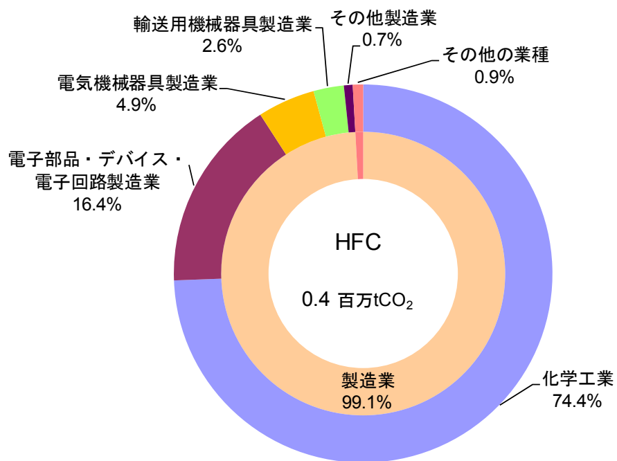
図 3-2 1 HFC【特定事業所】
