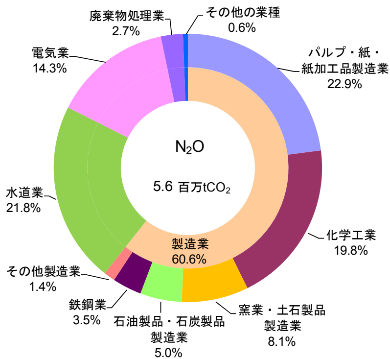
図 3 - 2 0 N 2 O【特定事業所】
