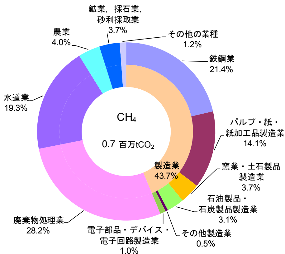
図 3 - 1 9 CH 4 【特定事業所】
