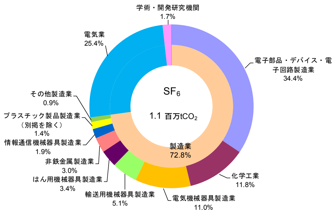
図 3-1 2 SF 6 【特定事業所排出者】
