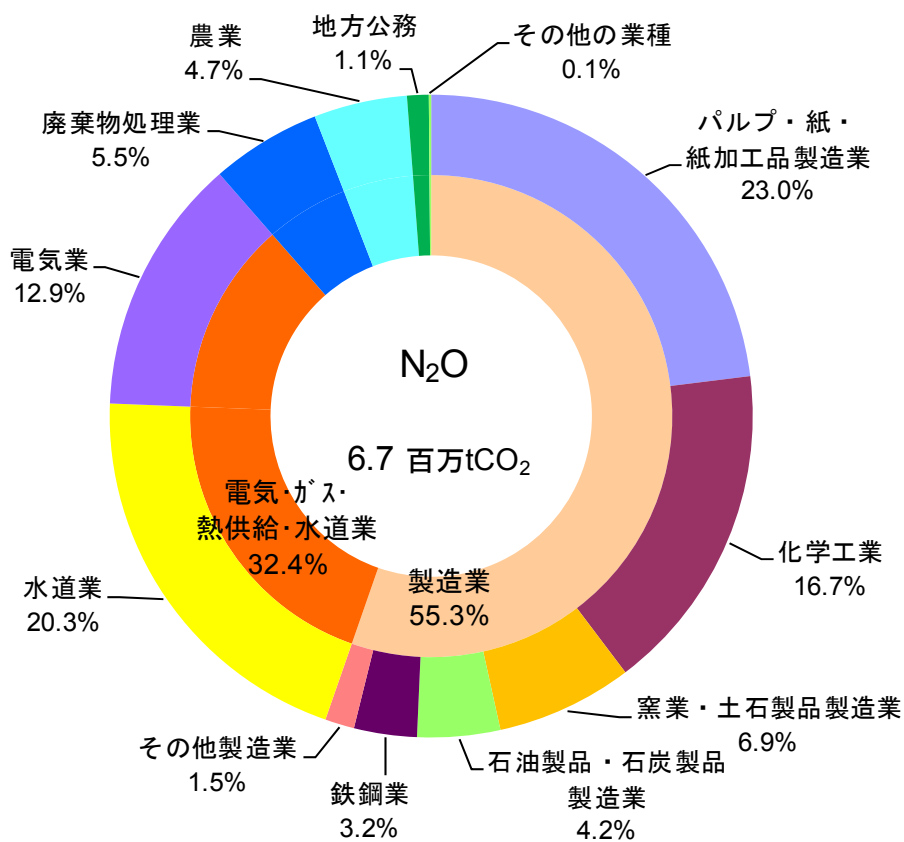
図 3-9 N 2 O【特定事業所排出者】
