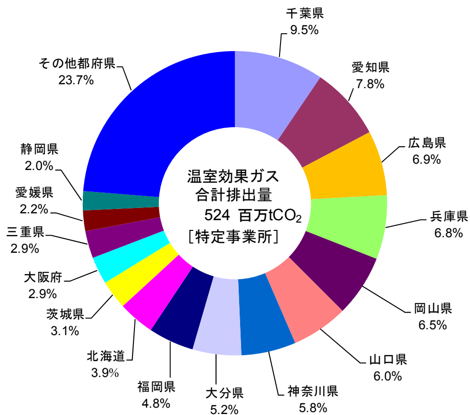
図 3-2 9 都道府県別の算定排出量【特定事業所】
