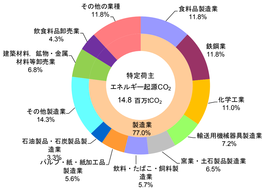
図 3-28 業種別の算定排出量【特定荷主】
