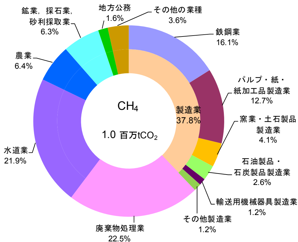
図 3-8 CH 4 【特定事業所排出者】
