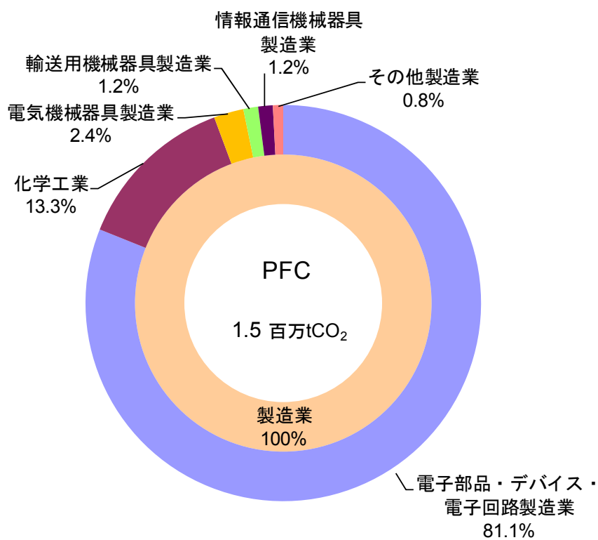
図 3-2 2 PFC【特定事業所】
