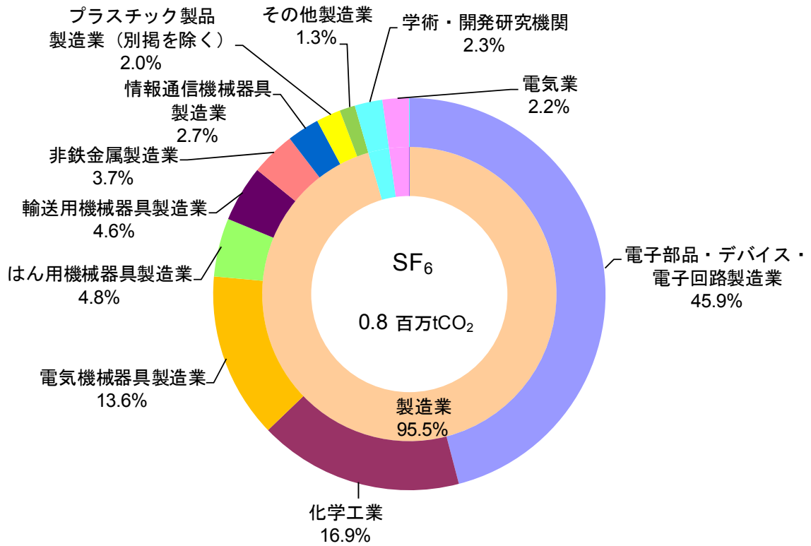
図 3-2 3 SF 6 【特定事業所】
