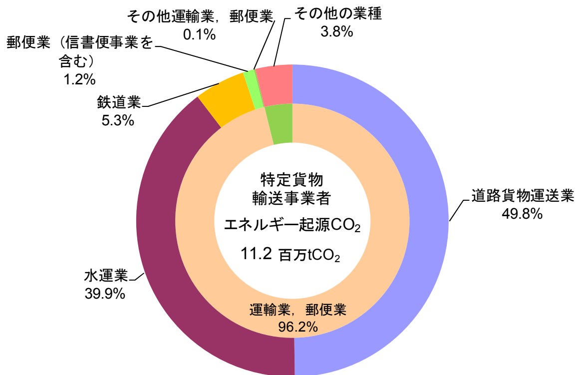
図 3-2 6 業種別の算定排出量【特定貨物輸送事業者】
