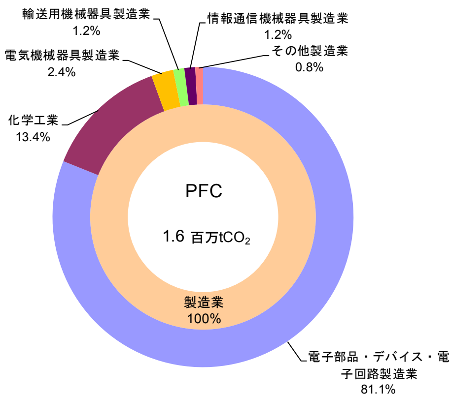
図 3 - 1 1 PFC【特定事業所排出者】
