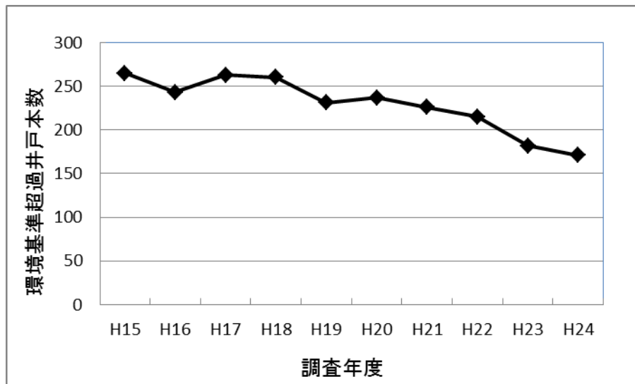
図6 地下水におけるトリクロロエチレンの環境基準 1 超過井戸本数の推移
