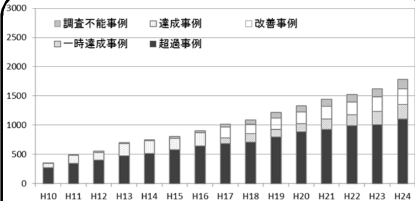
重金属等による汚染事例数の推移
