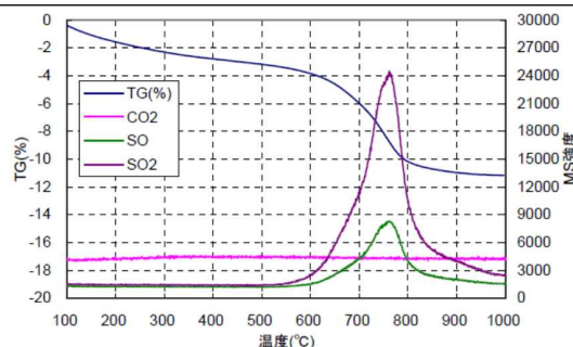
前段酸化触媒のTG/MS分析結果の一例 (600℃超でSO、SO 2 のピークが始まる。)
