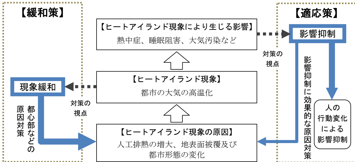
図1 ヒートアイランド現象に対する緩和策・適応策の概念図
