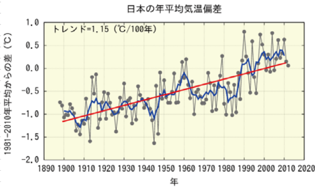
日本の年平均気温の変化 (1981～2010年平均からの偏差) 都市化の影響が比較的少ないとみられる17地点を用いた。黒線は年偏差、青線は5年移動平均、赤線は長期変化傾向。 出典4より
