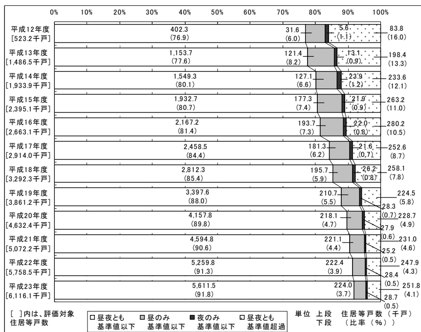
図8 環境基準の達成状況の評価結果（全国・経年変化）
