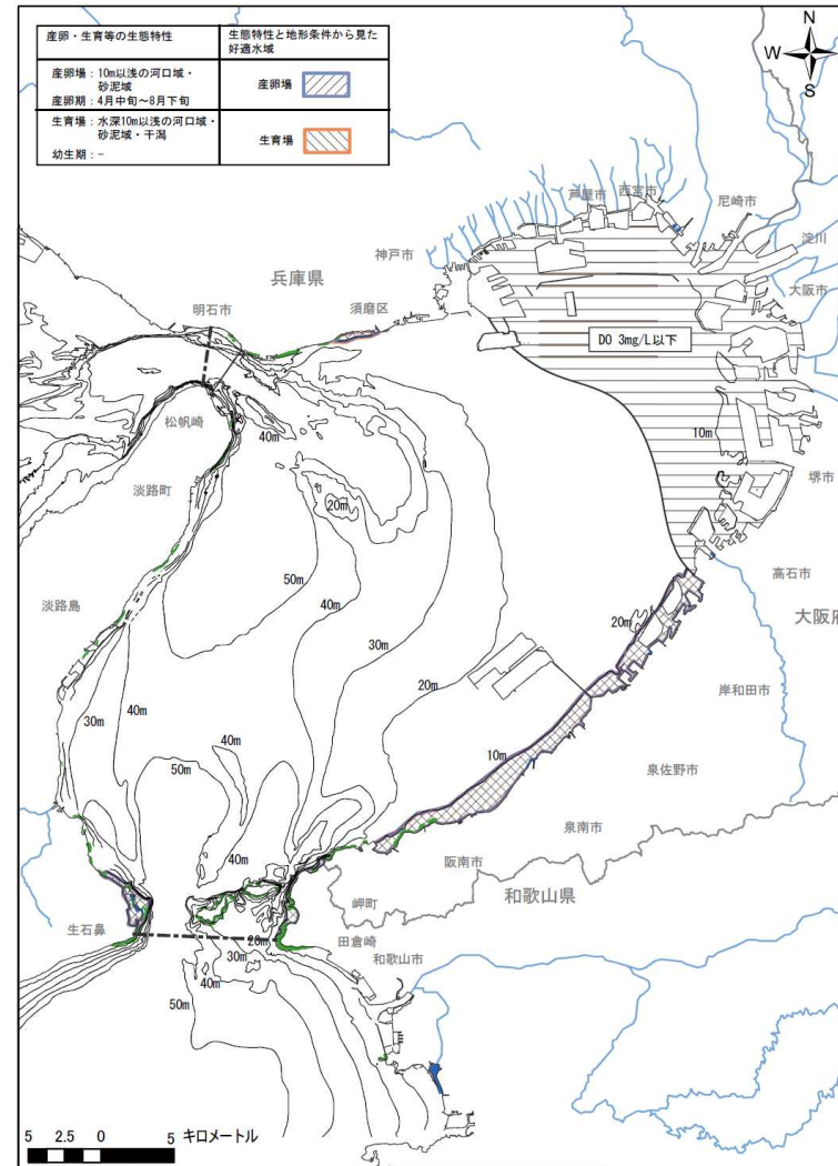
大阪湾 生態特性、地理条件及び水域条件からみた好適な水域 【魚種：ガザミ（産卵場）（生育場）（DO好適水域）】
