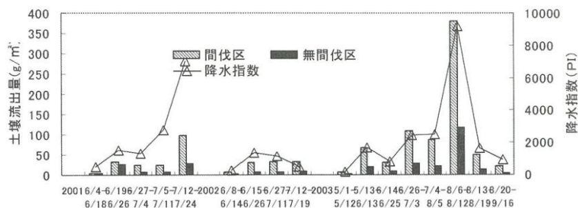
間伐区と無間伐区の土砂流出量の比較 (ヒノキ林 定性間伐) (出典) 手島志穂: 間伐の推進にかかる施業効果の総合評価に関する研究, 大分県林業試験場年報, No.46, p22-25 (2004)
