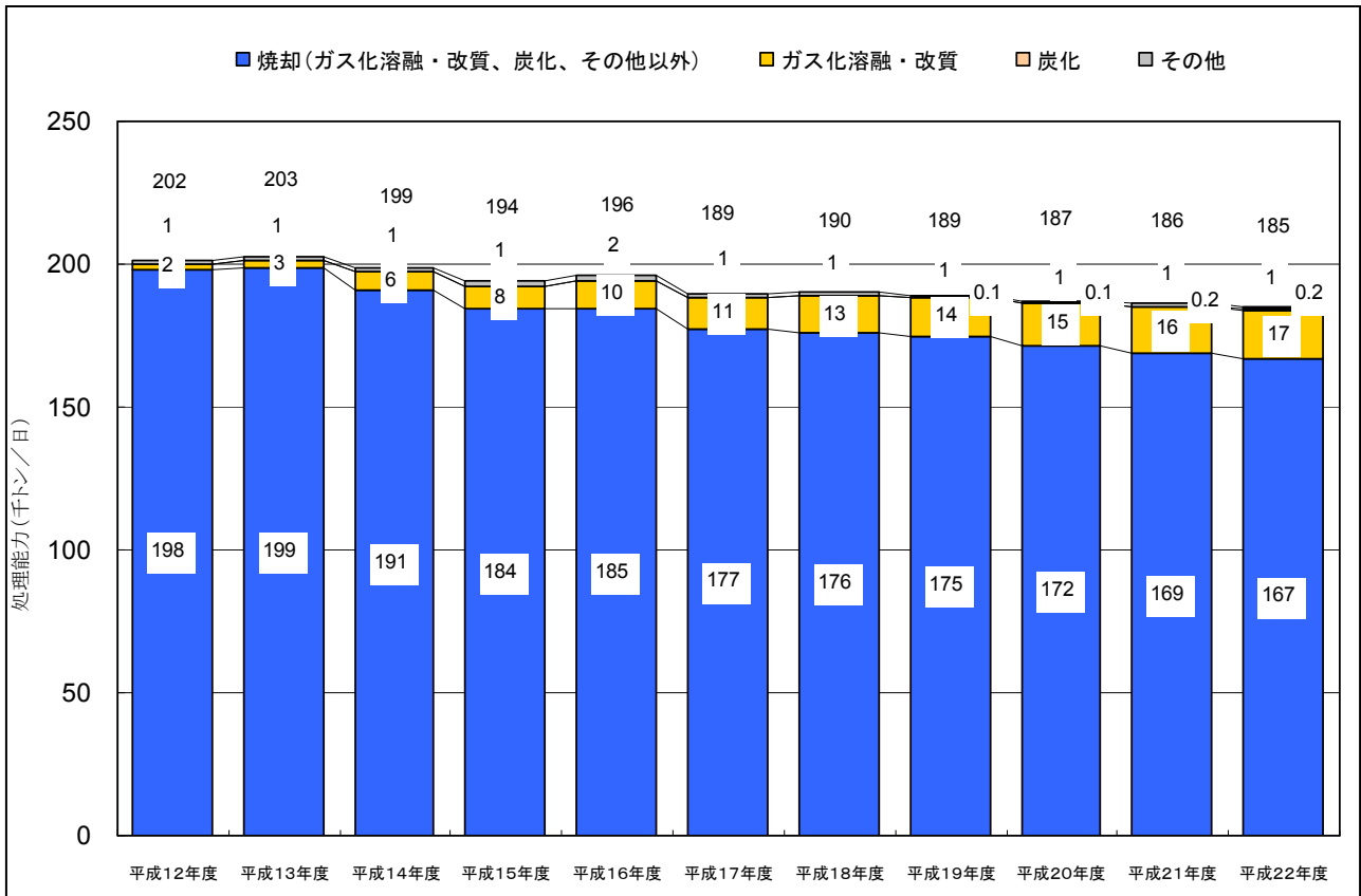
図-10 ごみ焼却施設の種別処理能力の推移
