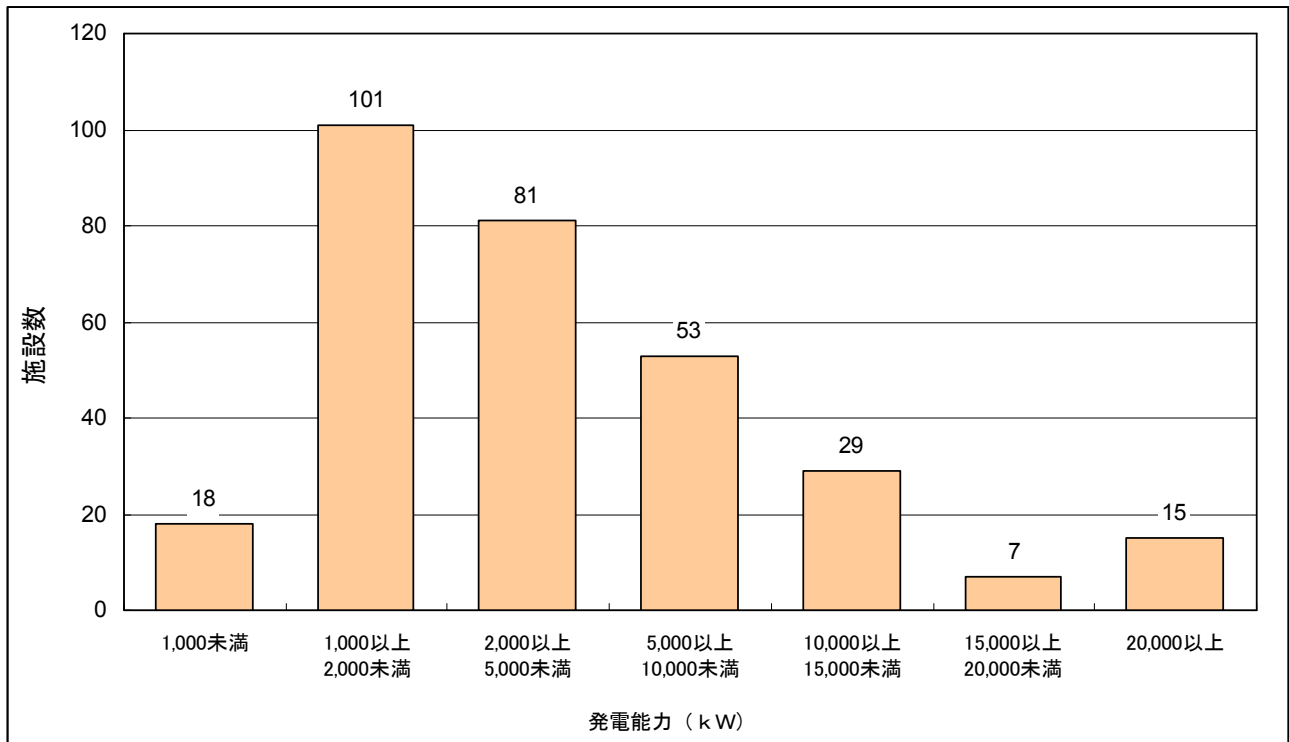
図-15 ごみ焼却施設の発電能力別の施設数
