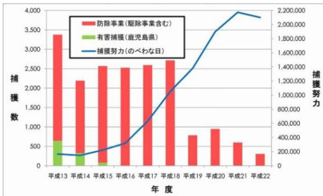
図２－４ 奄美大島におけるジャワマングースの捕獲頭数及び捕獲努力の経年変化（環境省による防除）
