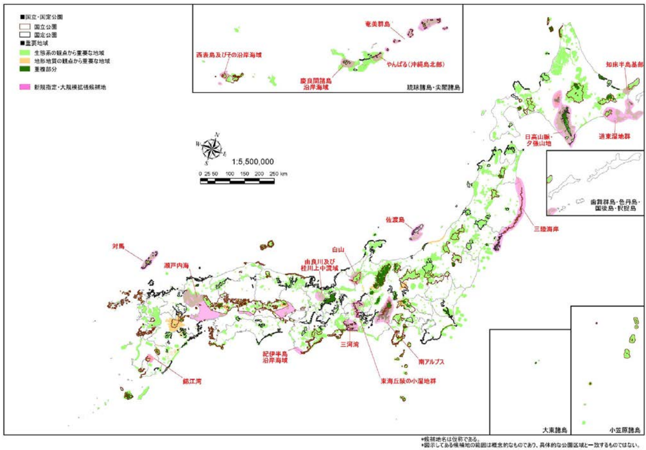
図3-1 生態系・地形地質の観点から重要な地域の分布と新規指定・大規模拡張候補地〔全国〕
