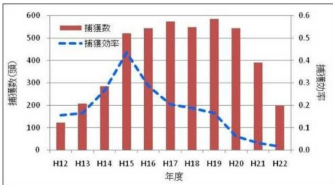
図２－５ 沖縄県北部地域（やんばる）におけるジャワマングースの捕獲頭数と捕獲効率の経年変化（環境省と沖縄県による防除）
