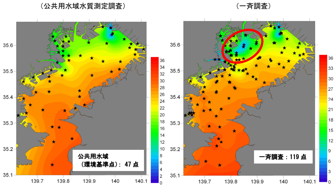
図 1 表層塩分の水平分布の比較
